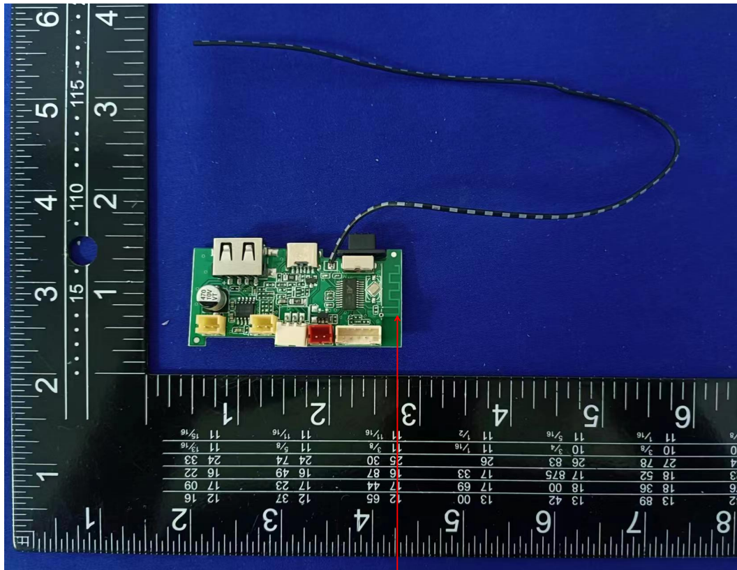
PCB ANT
