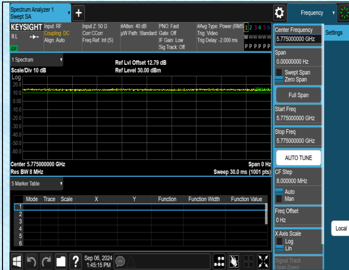
NTNV-11AC80SISO-Ant3-5775
