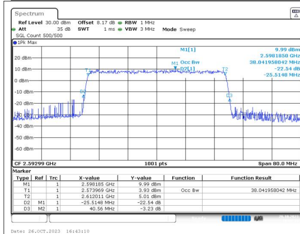
n41 SCS=30kHz CP_QAM256 BW=40MHz Channel=518598 RB=106@0
