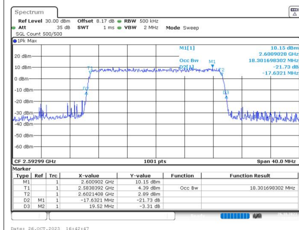
n41 SCS=30kHz CP_QAM256 BW=20MHz Channel=518598 RB=51@0
