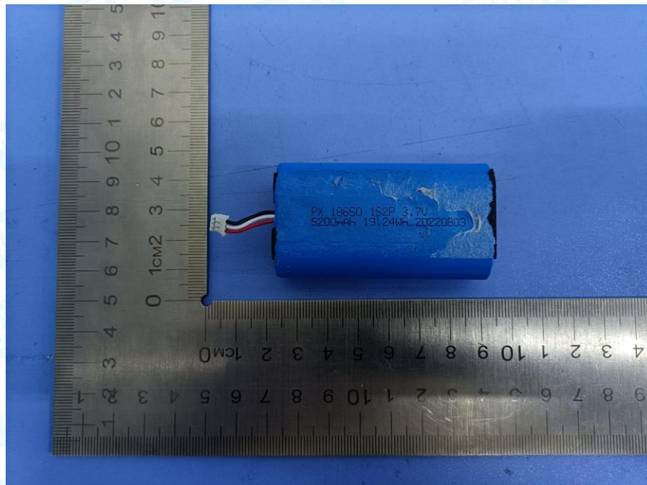
Photo 10 Battery parameters
