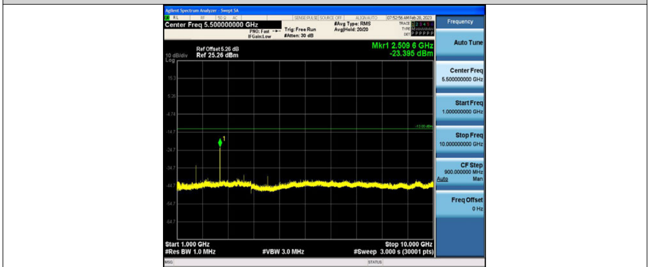
GPRS850-190-1000~10000MHz
