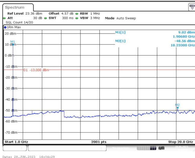
Band2-9538-3-1000~20000MHz
