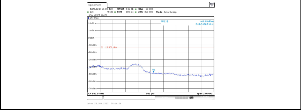
Band5-3MHz-QPSK-20635-1RB#0
