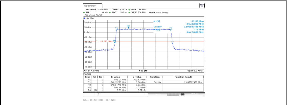
Band5-3MHz-QPSK-20635-15RB#0-2.696
