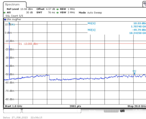
Band4-10MHz-QPSK-20000-1RB#0-Range4:1000~20000MHz
