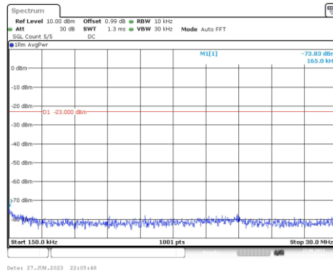
Band4-10MHz-QPSK-20000-1RB#0-Range2:0.15~30MHz
