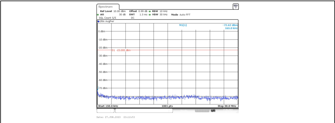
Band4-20MHz-QPSK-20175-1RB#0-Range2:0.15~30MHz
