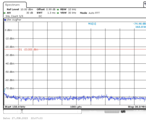
Band4-10MHz-QPSK-20175-1RB#0-Range2:0.15~30MHz
