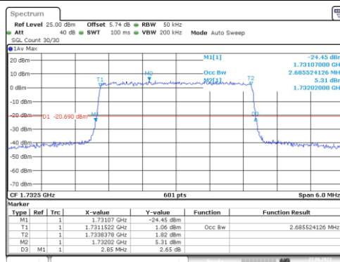
Band4-3MHz-OPSK-20175-15RB#0-2.686
