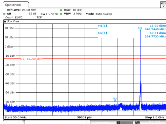
Band5_3MHz_QPSK_20635_1RB#14
