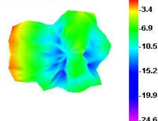
5850.000MHz
