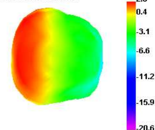
2480.000MHz
