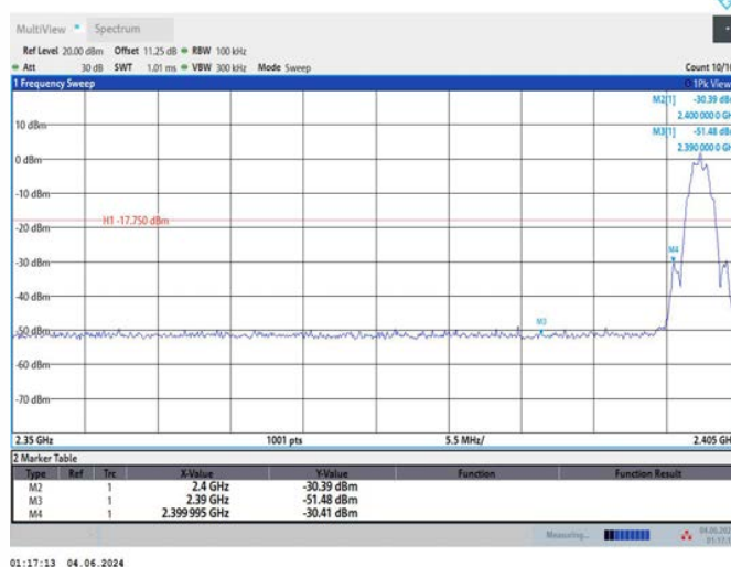
BLE_2M_Ant1_Low_2402
