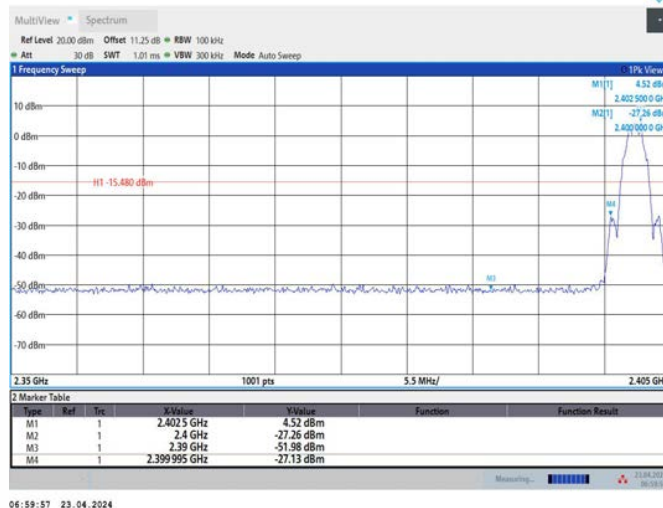
BLE_2M_Ant1_Low_2402
