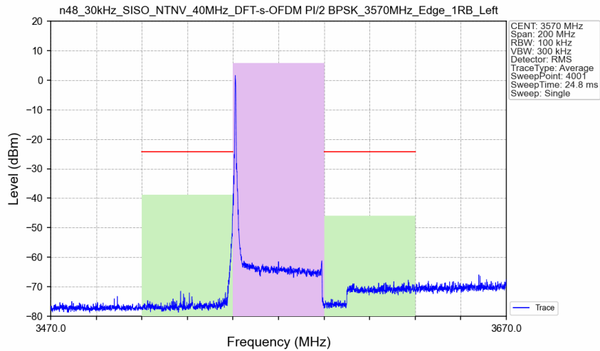
n48_30kHz_SISO_NTNV_40MHz_DFT-s-OFDM PI/2 BPSK_3570MHz_Edge_1RB_Left_Ant3
