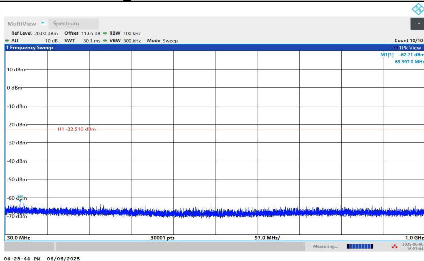
BLE_2M-Ant1-2480-30~1000-PASS
