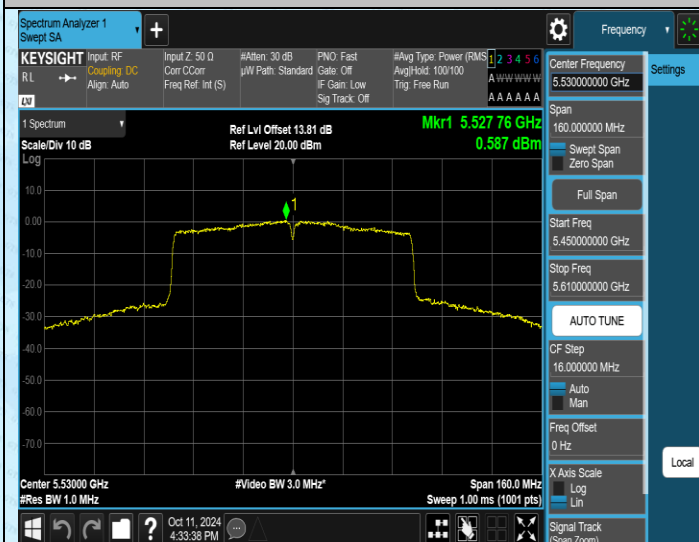
11AC80SISO-Ant1-5530-PASS
