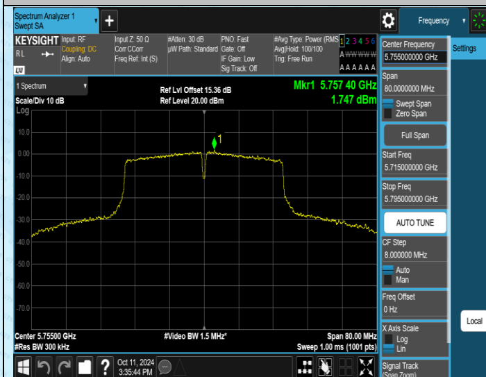
11N40SISO-Ant1-5755-PASS
