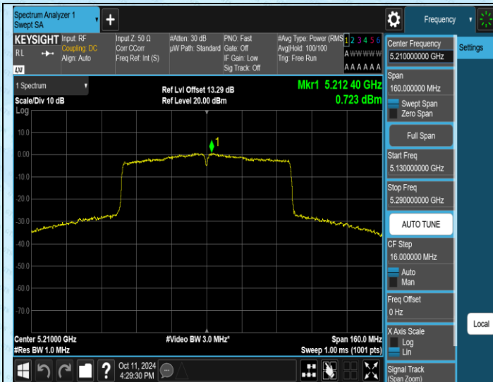
11AC80SISO-Ant1-5210-PASS
