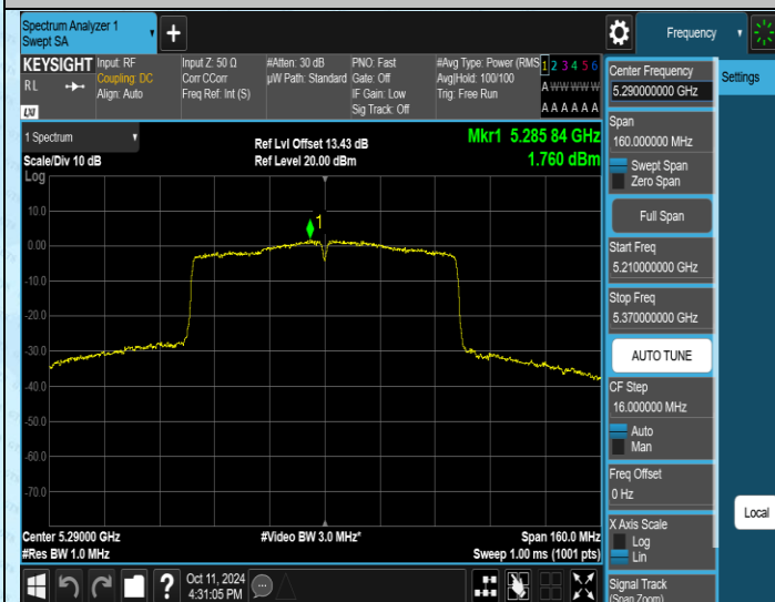
11AC80SISO-Ant1-5290-PASS
