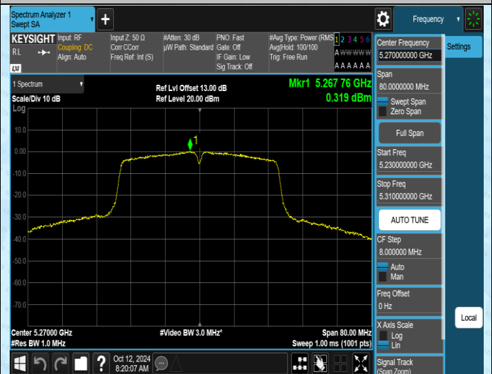
11N40SISO-Ant2-5270-PASS
