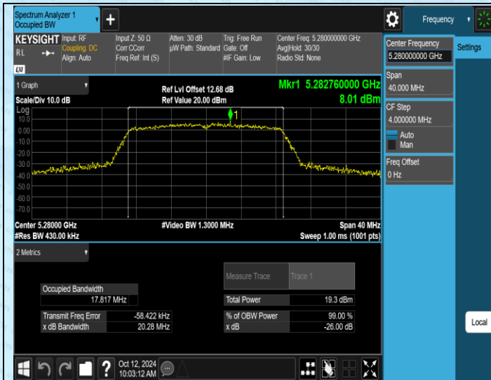
11N20MIMO-Ant1-5280
