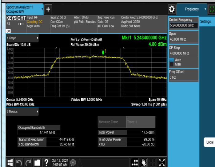
11N20MIMO-Ant1-5240
