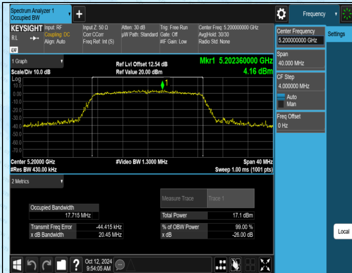
11N20MIMO-Ant1-5200
