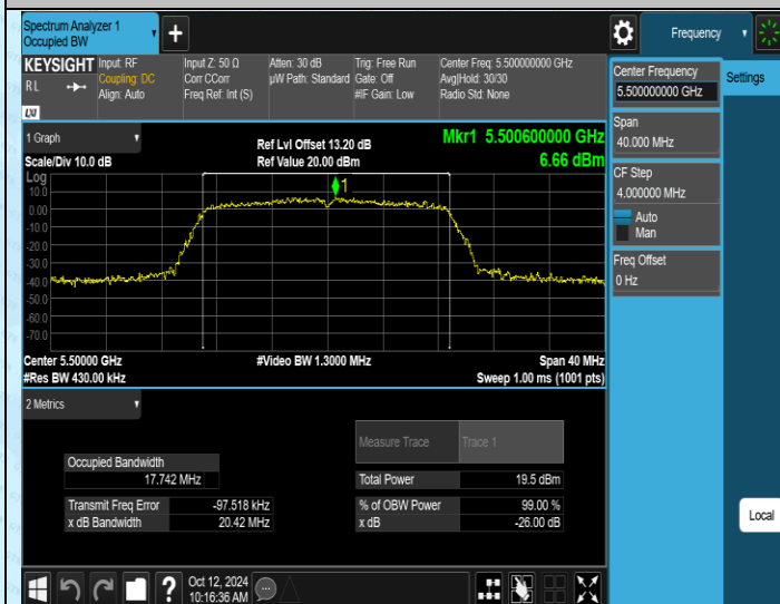
11N20MIMO-Ant1-5500
