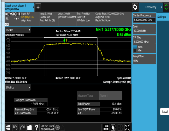
11N20MIMO-Ant1-5320
