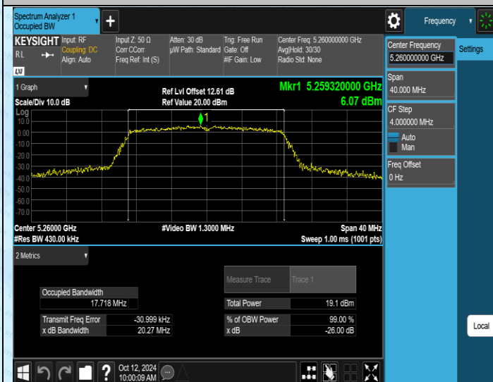
11N20MIMO-Ant1-5260
