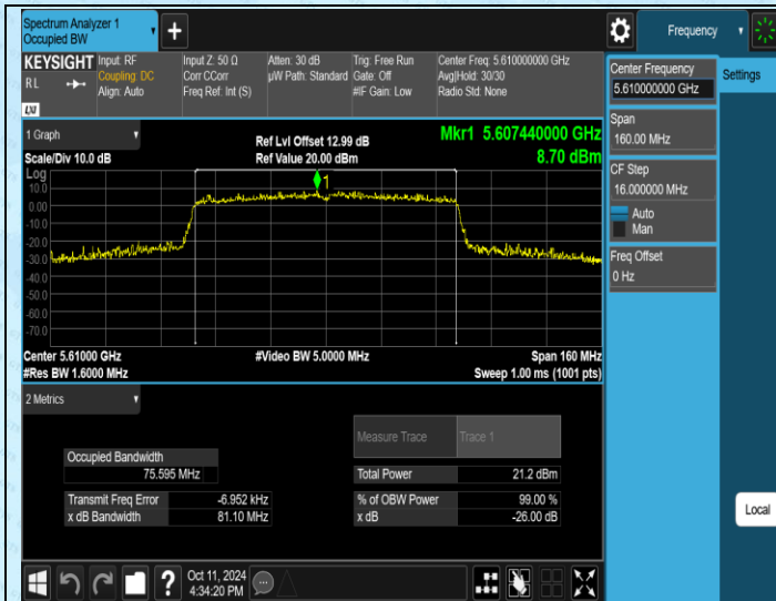
11AC80SISO-Ant1-5610
