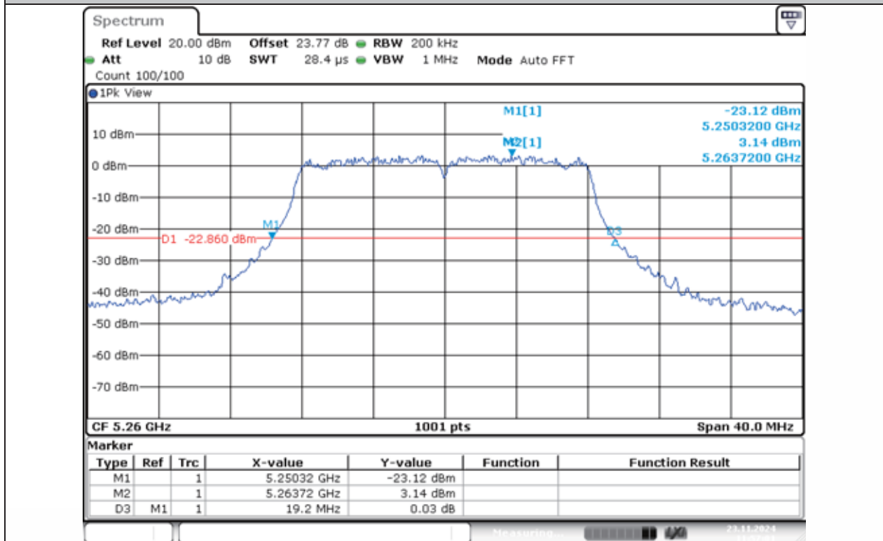
11A-Ant1-5260
