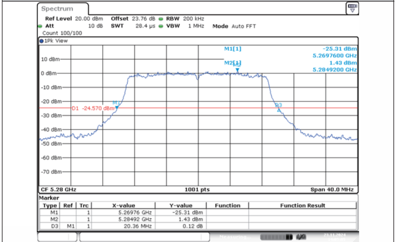
11N20MIMO-Ant1-5280
