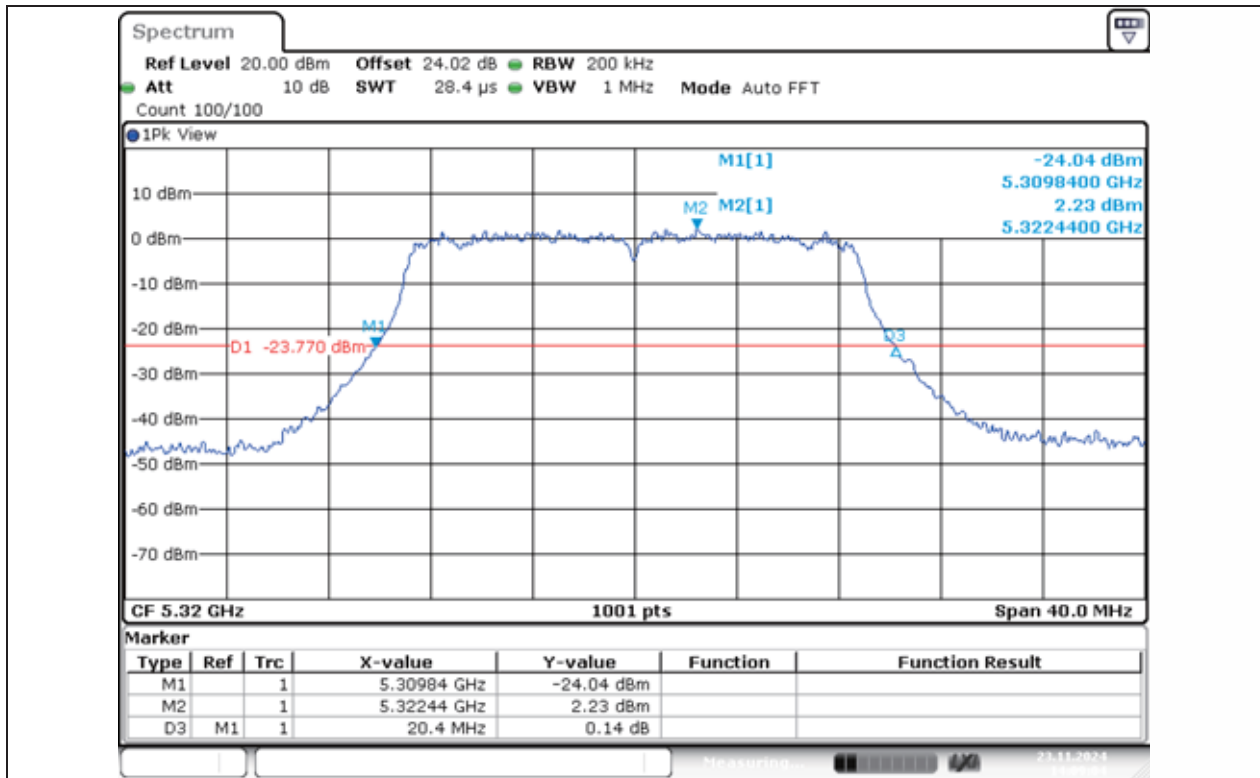
11N20MIMO-Ant1-5320
