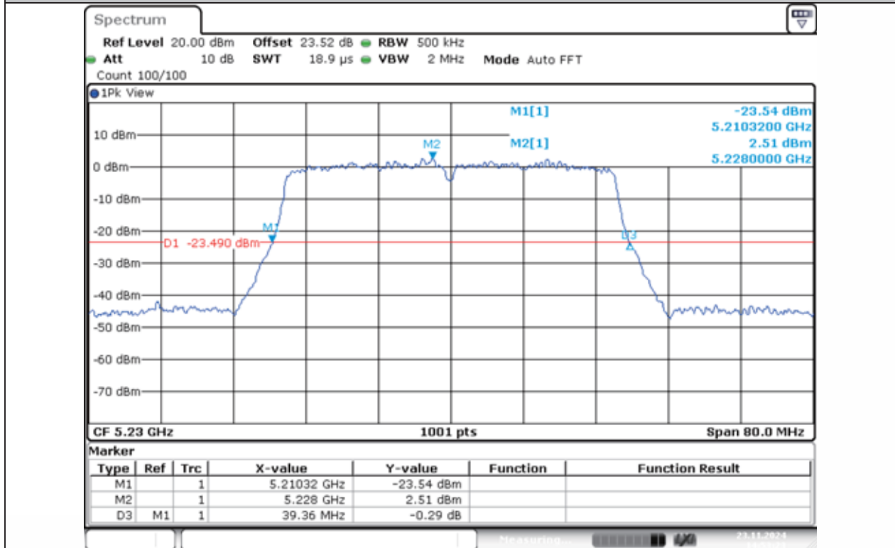
11N40MIMO-Ant1-5230
