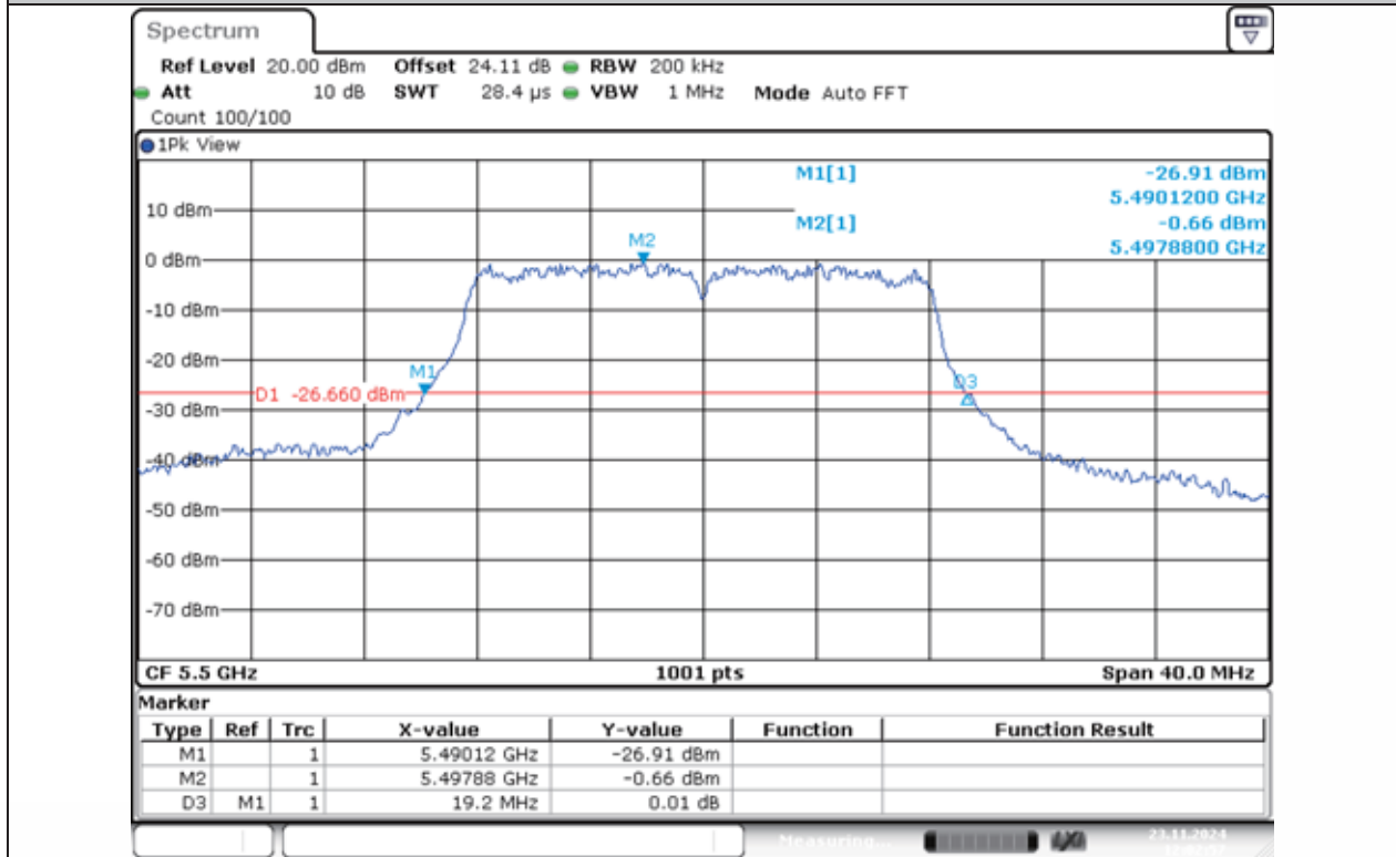
11A-Ant1-5500
