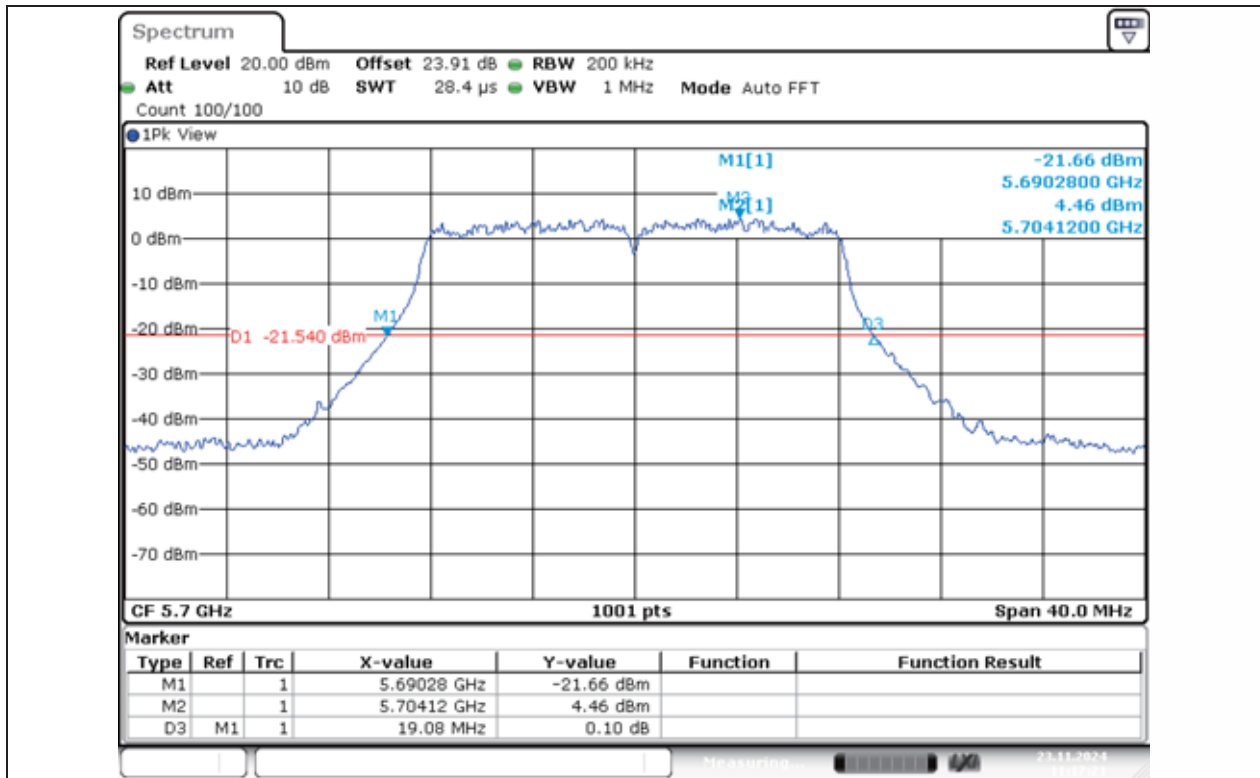
11A-Ant1-5700
