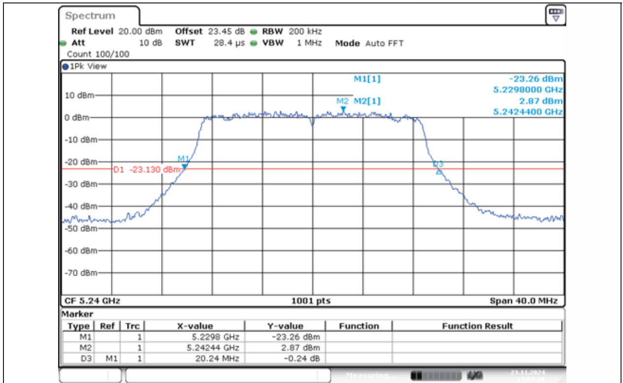
11N20MIMO-Ant1-5240
