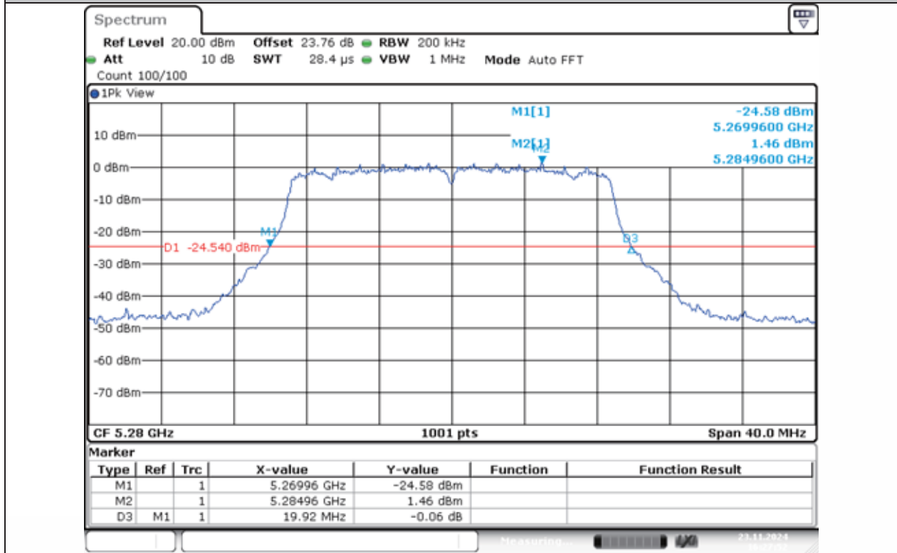
11AC20MIMO-Ant1-5280
