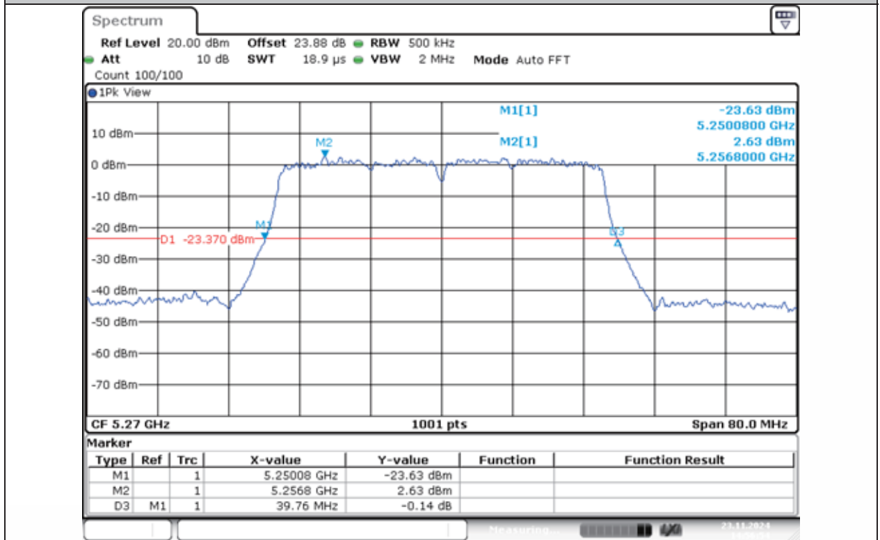
11N40MIMO-Ant1-5270
