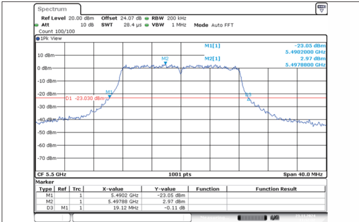
11A-Ant1-5500
