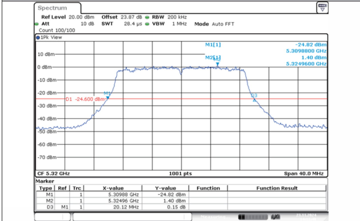
11N20MIMO-Ant1-5320
