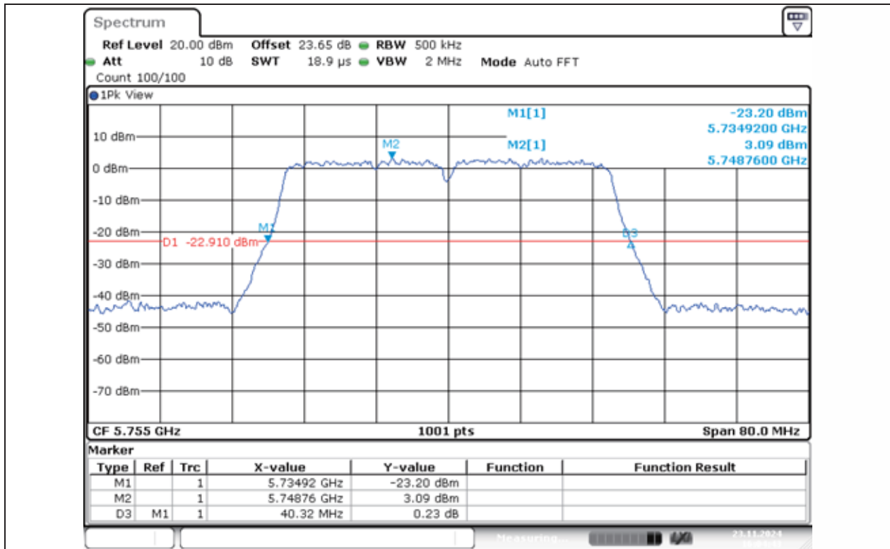
11N40MIMO-Ant1-5755
