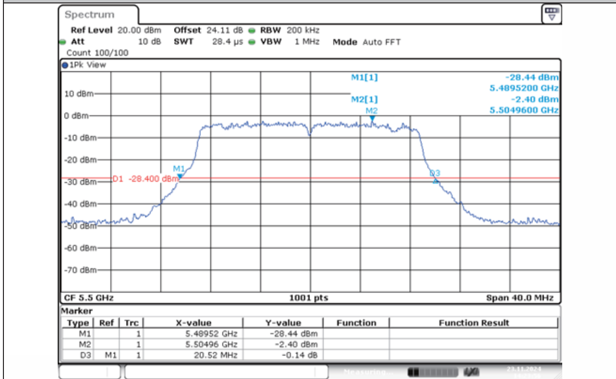
11N20MIMO-Ant1-5500
