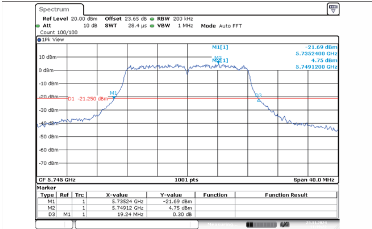
11A-Ant1-5745
