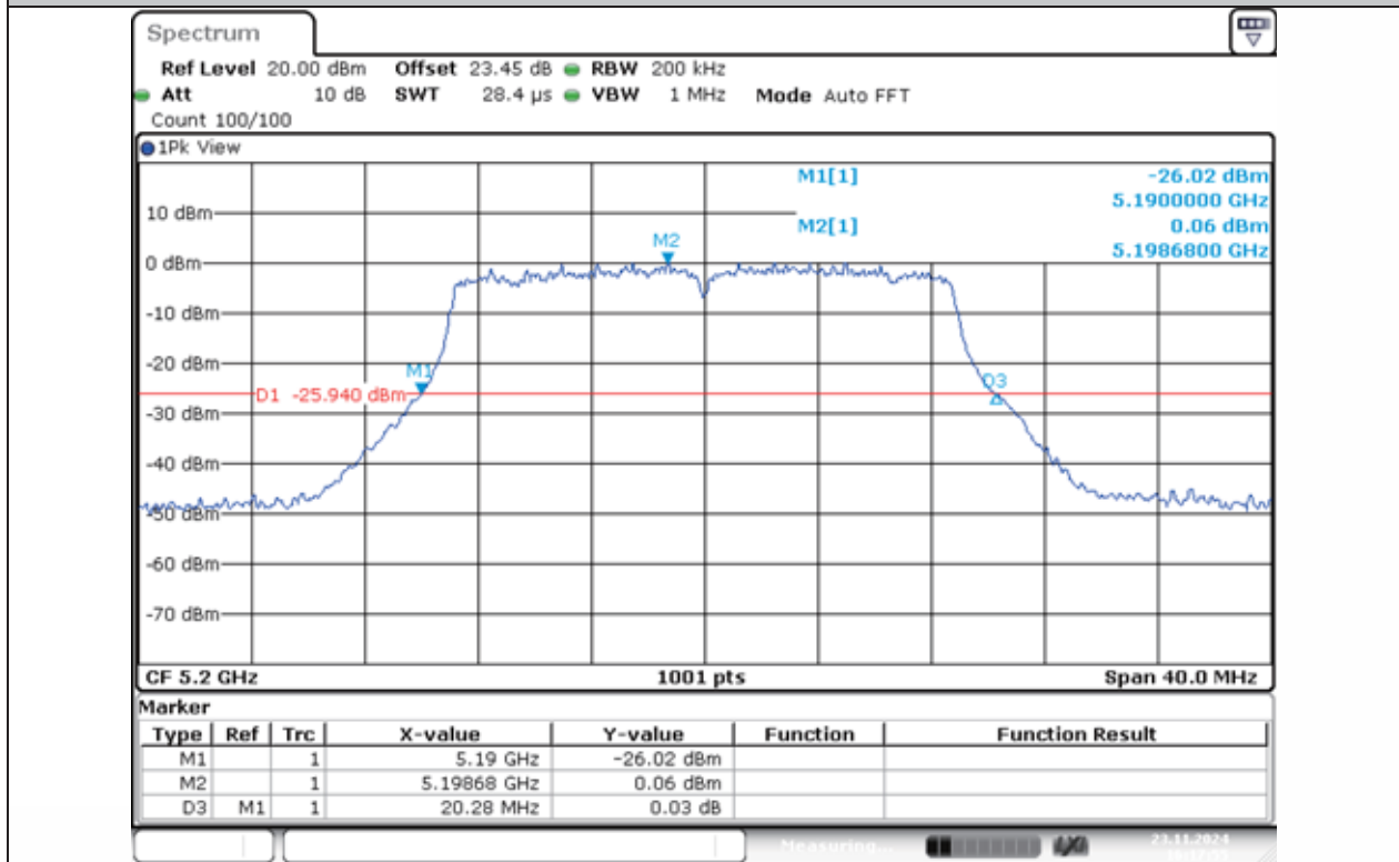
11AC20MIMO-Ant1-5200
