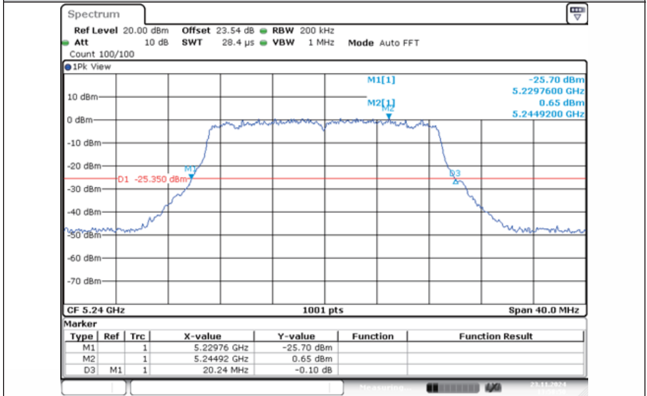
11N20MIMO-Ant1-5240
