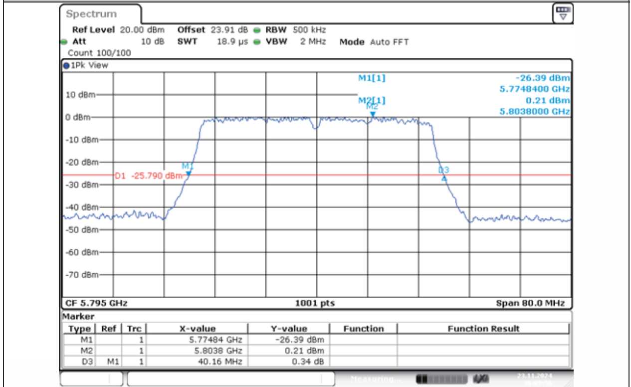
11N40MIMO-Ant1-5795
