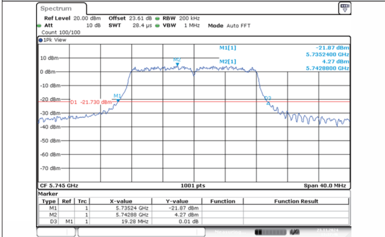
11A-Ant1-5745
