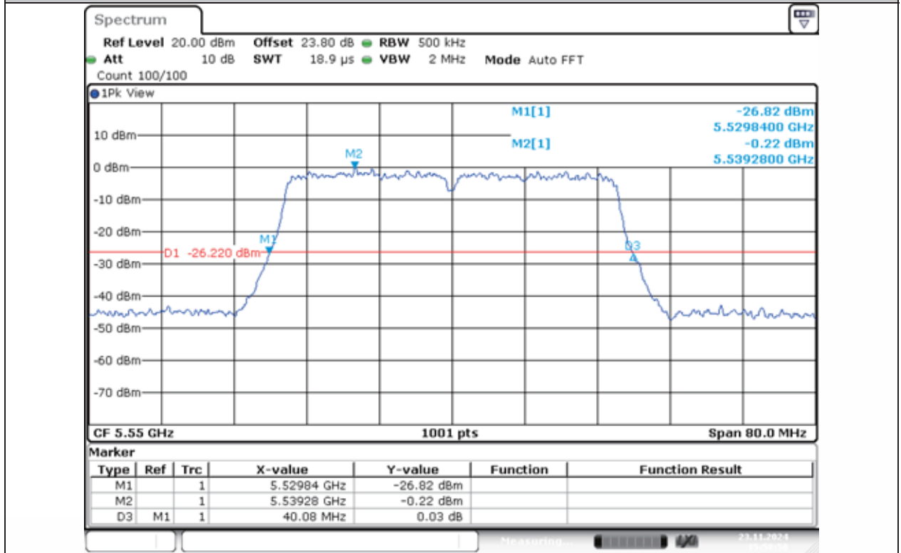
11N40MIMO-Ant1-5550
