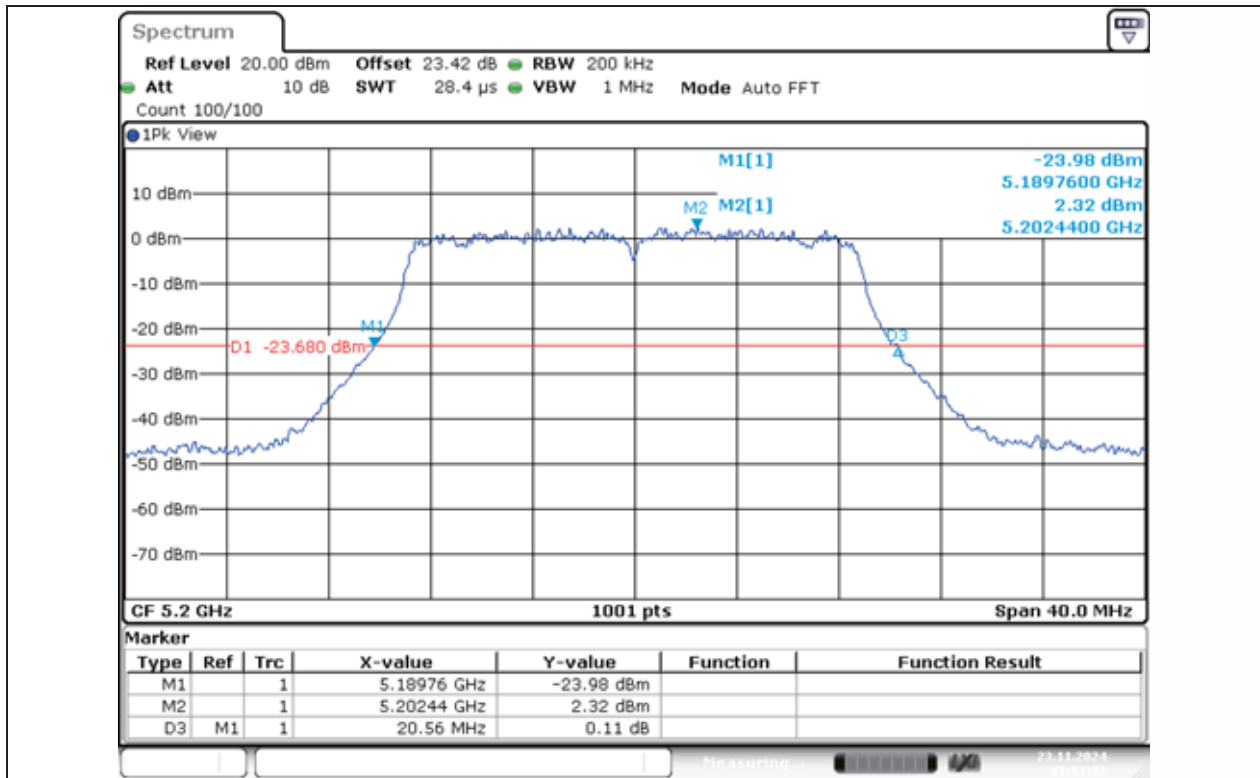
11N20MIMO-Ant1-5200
