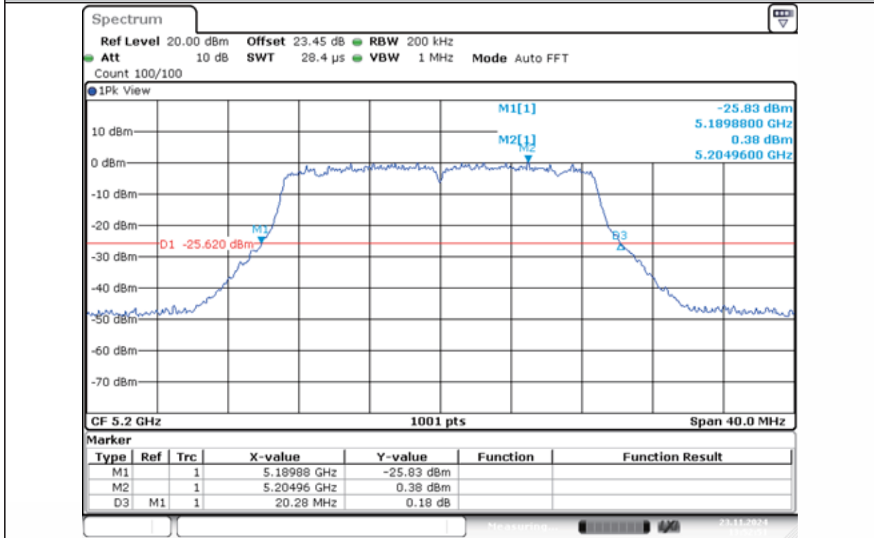
11N20MIMO-Ant1-5200
