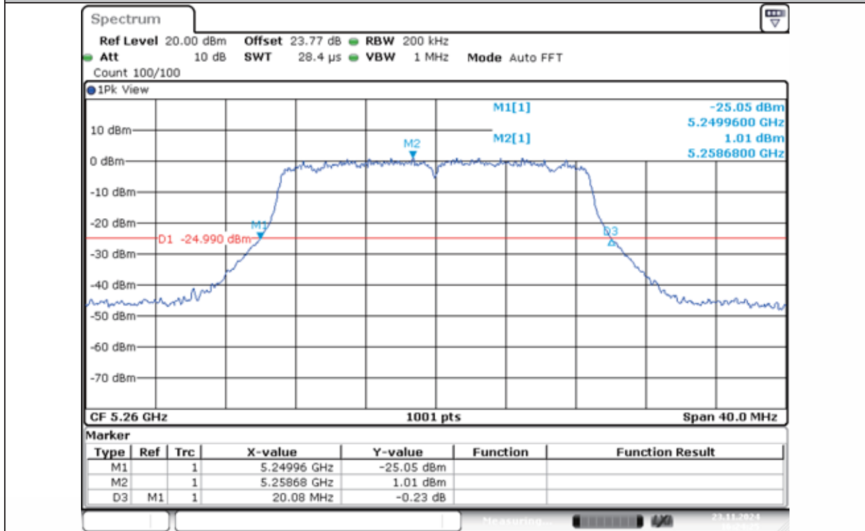
11AC20MIMO-Ant1-5260
