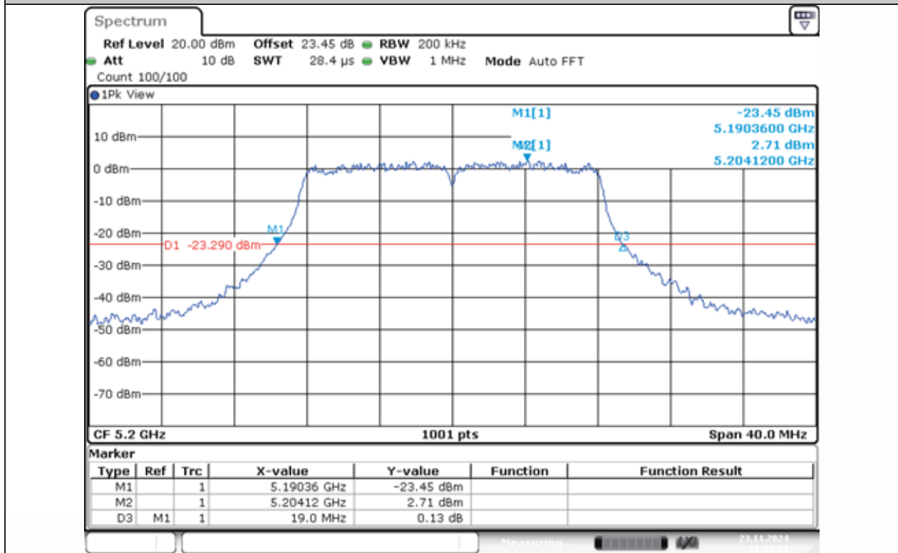
11A-Ant1-5200
