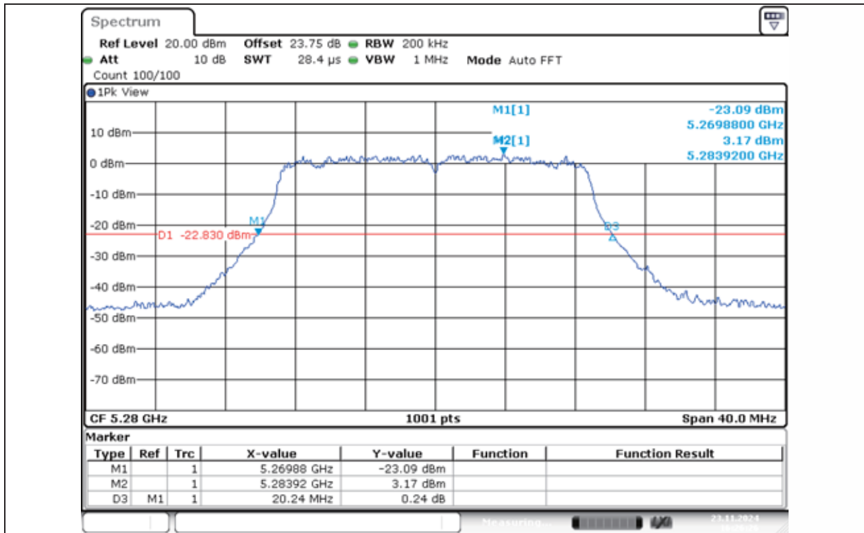
11AC20MIMO-Ant1-5280
