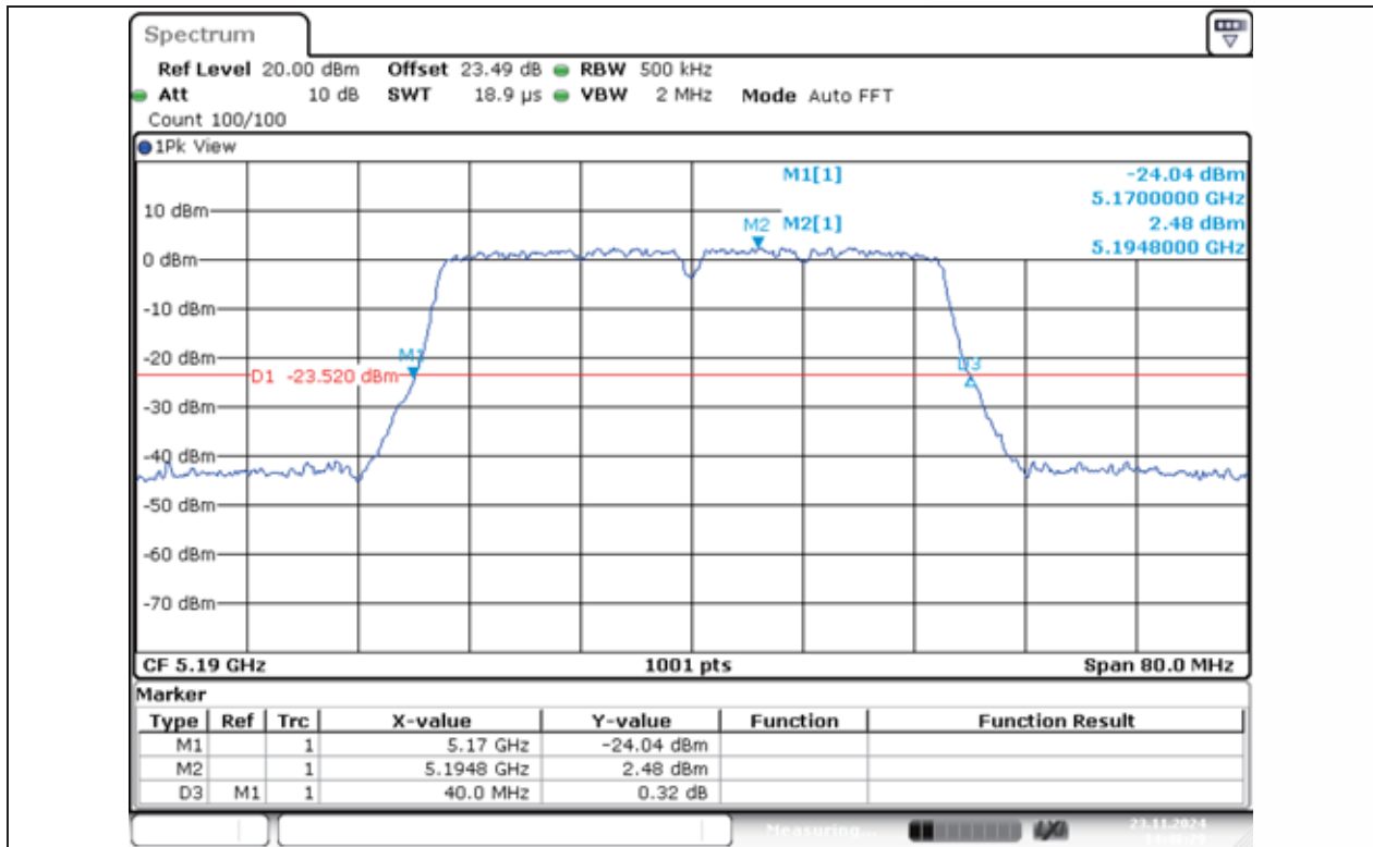
11N40MIMO-Ant1-5190
