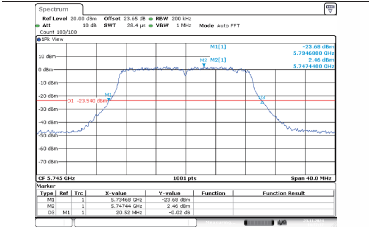
11N20MIMO-Ant1-5745
