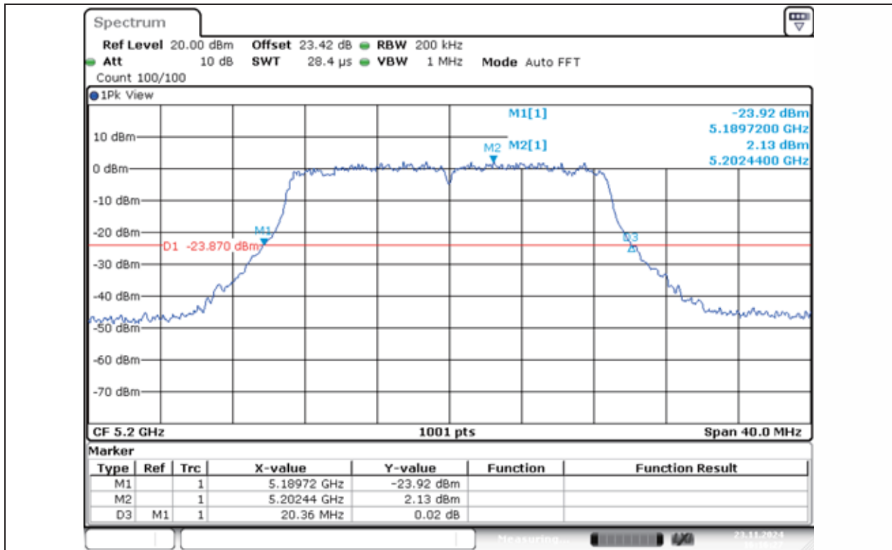
11AC20MIMO-Ant1-5200
