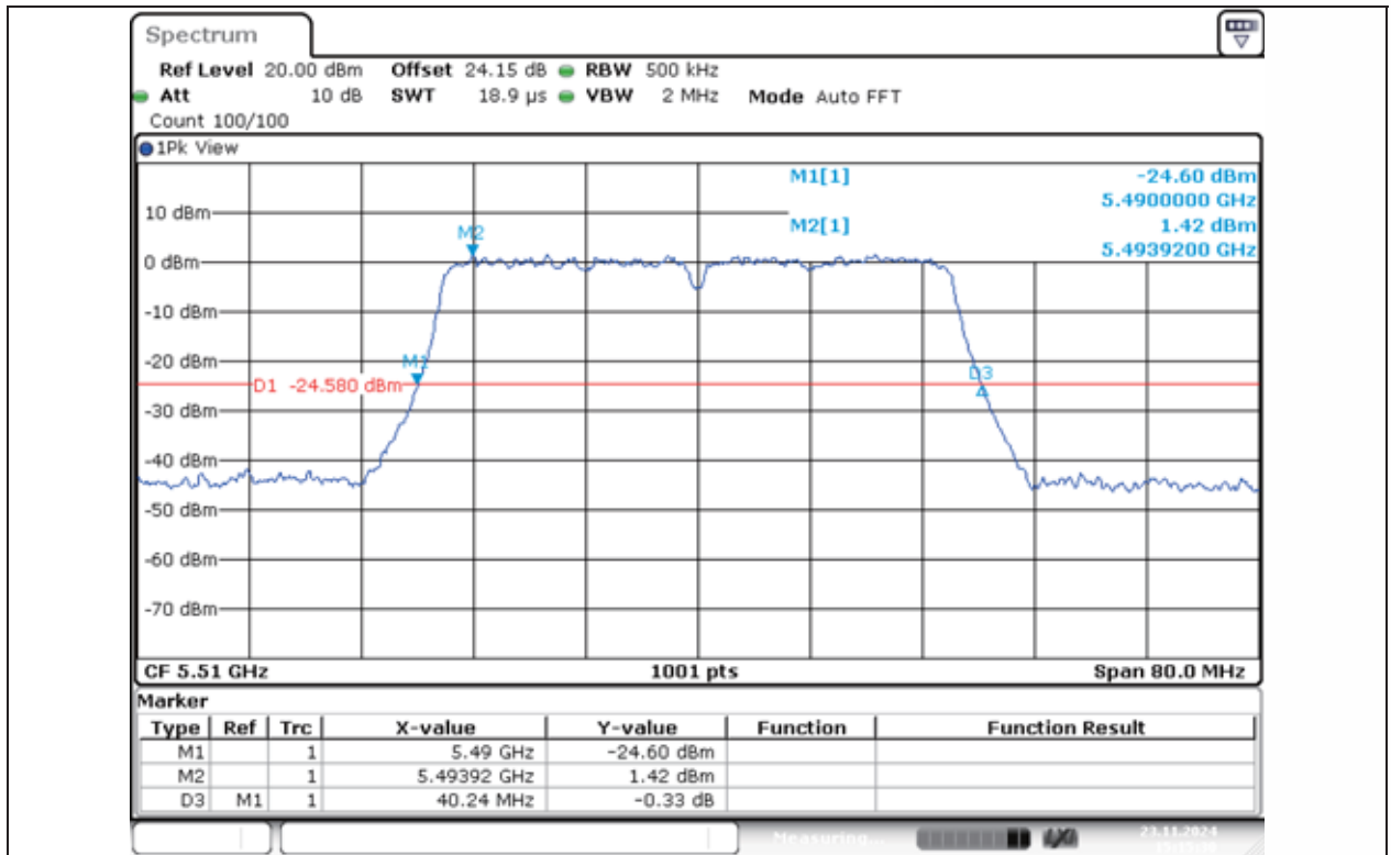
11N40MIMO-Ant1-5510
