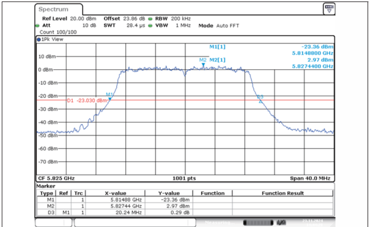
11N20MIMO-Ant1-5825
