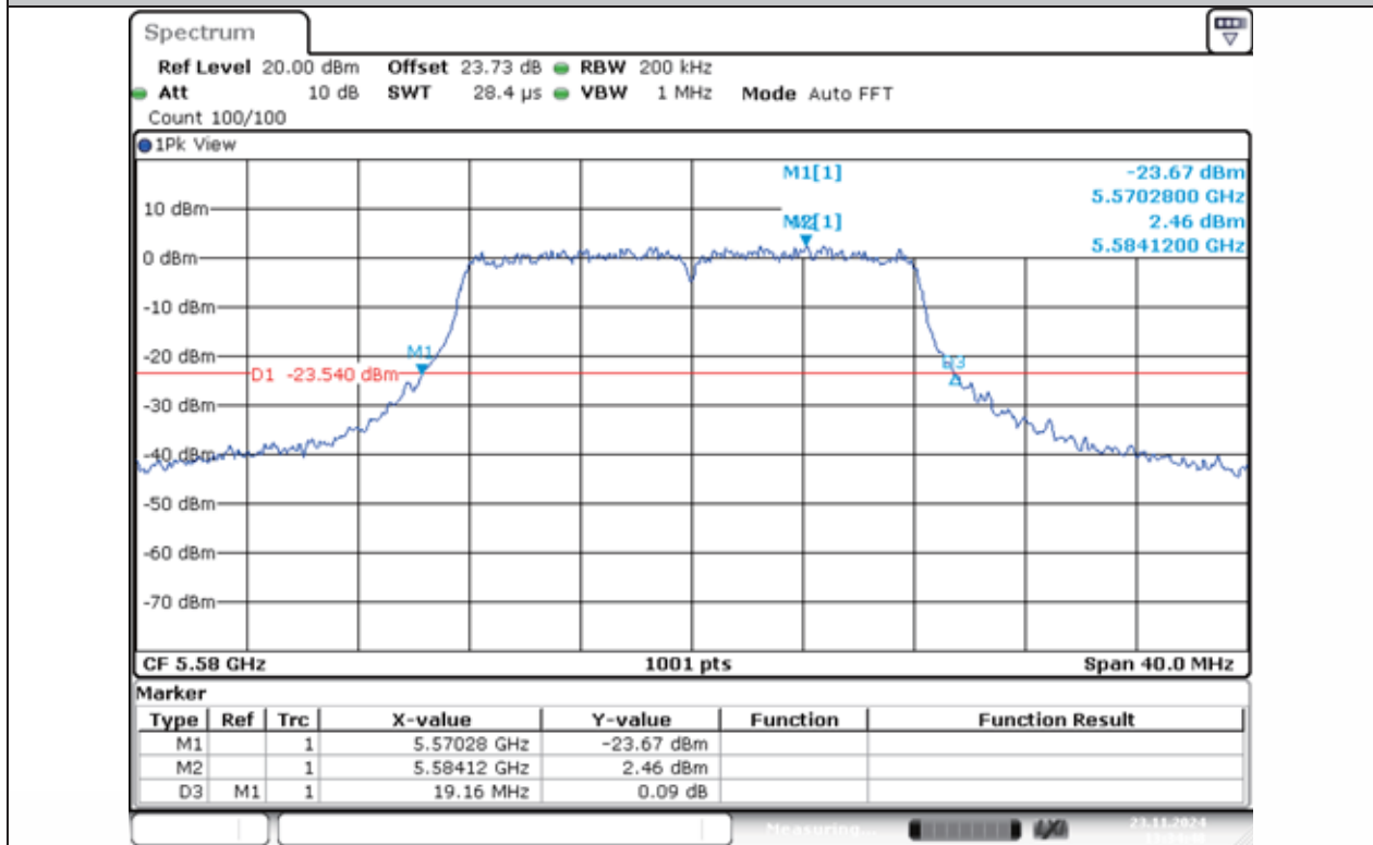
11A-Ant1-5580
