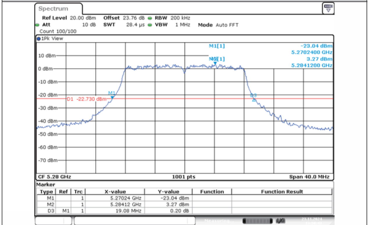
11A-Ant1-5280
