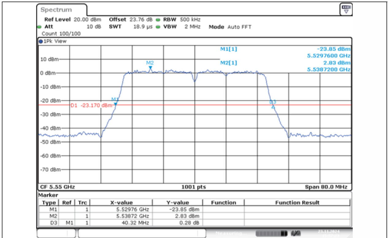
11N40MIMO-Ant1-5550
