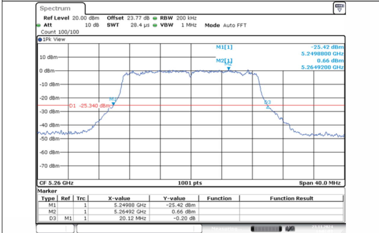
11N20MIMO-Ant1-5260
