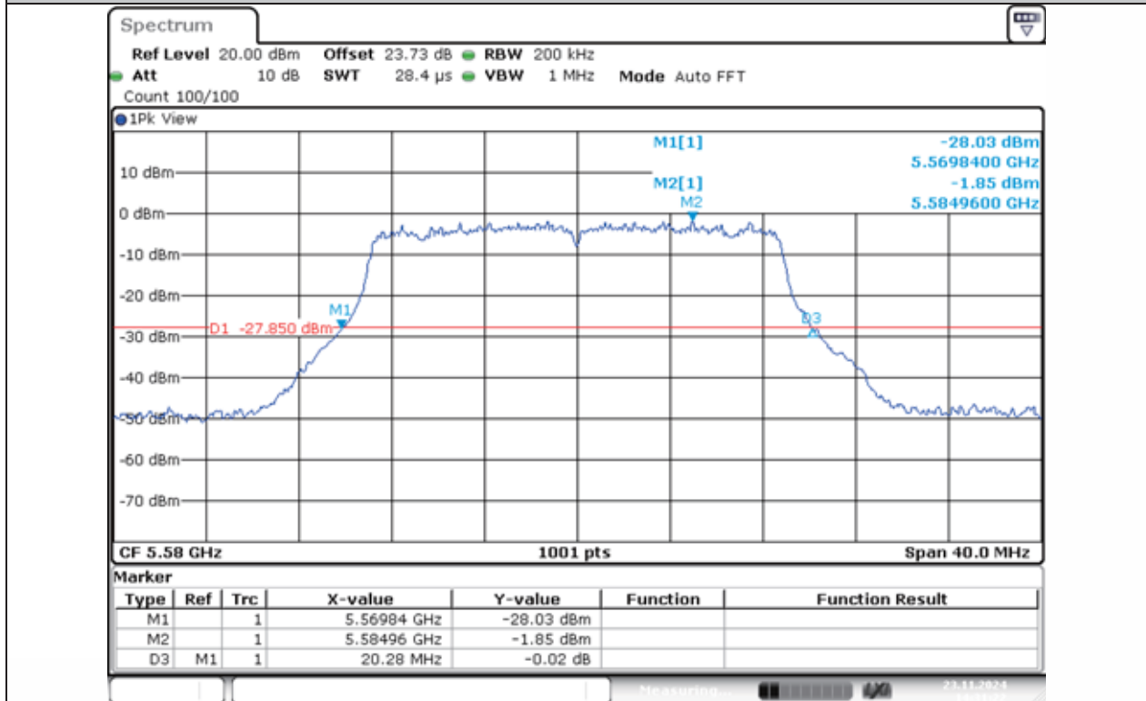
11N20MIMO-Ant1-5580
