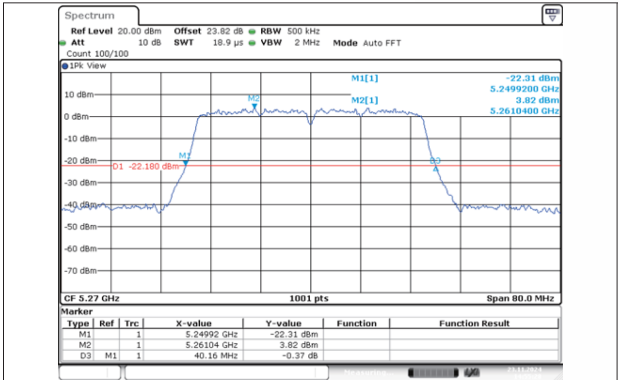
11N40MIMO-Ant1-5270
