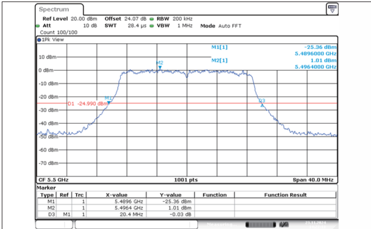
11N20MIMO-Ant1-5500
