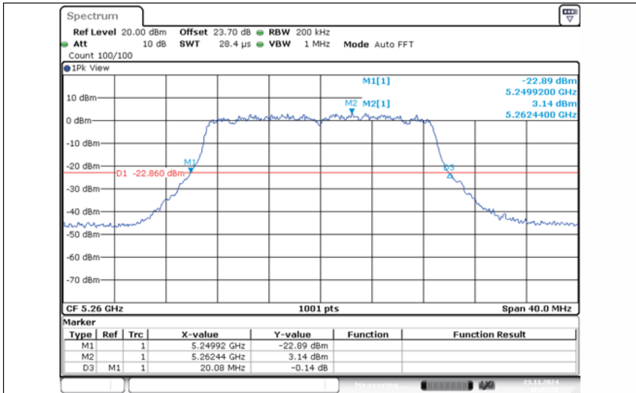
11AC20MIMO-Ant1-5260
