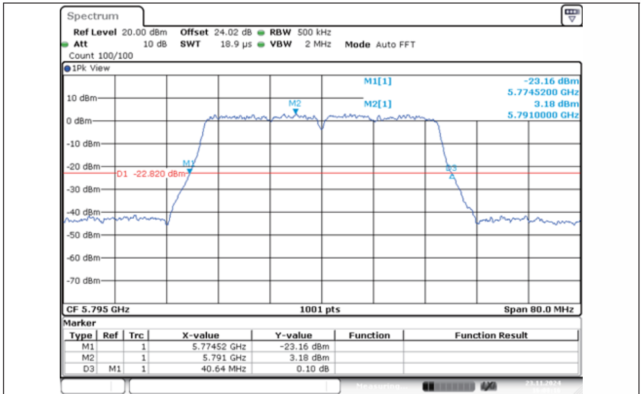
11N40MIMO-Ant1-5795
