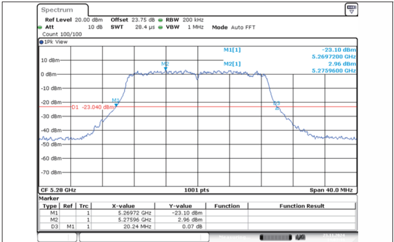
11N20MIMO-Ant1-5280
