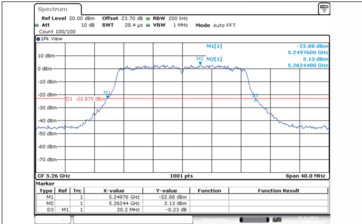
11N20MIMO-Ant1-5260
