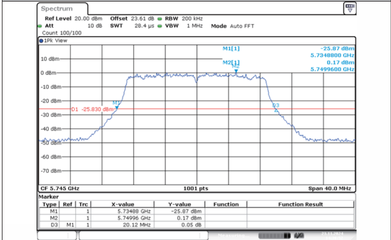
11N20MIMO-Ant1-5745
