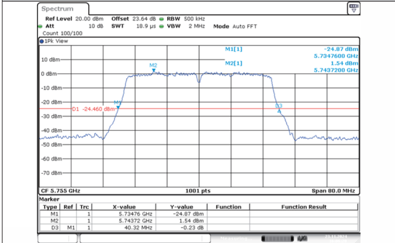
11N40MIMO-Ant1-5755
