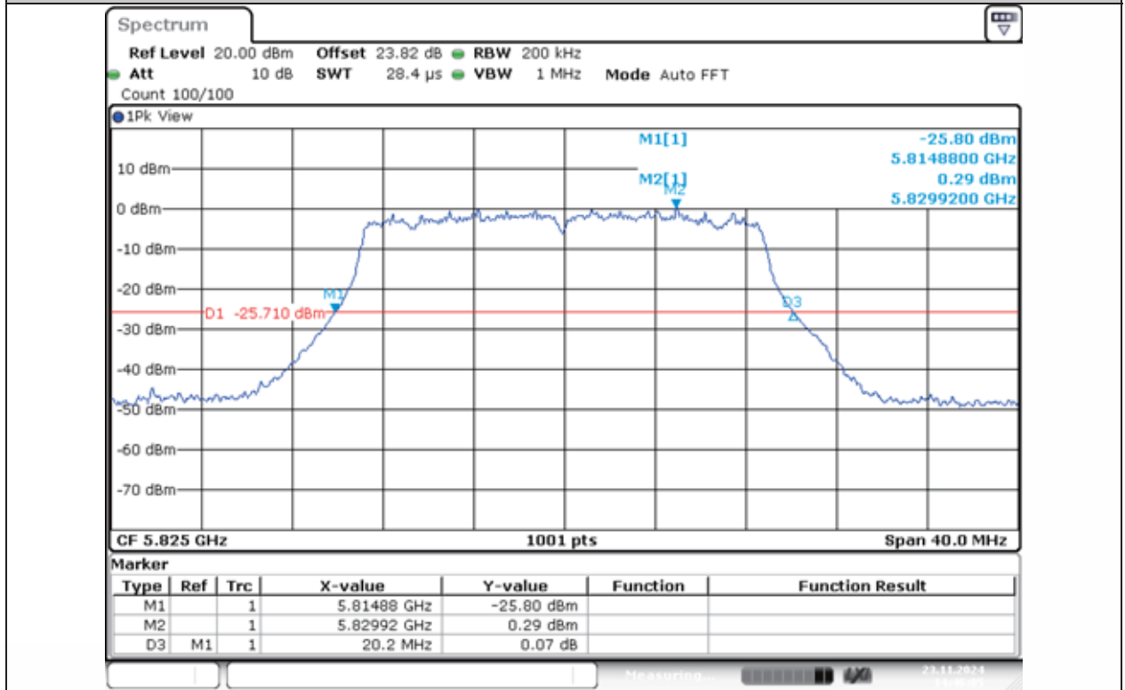
11N20MIMO-Ant1-5825
