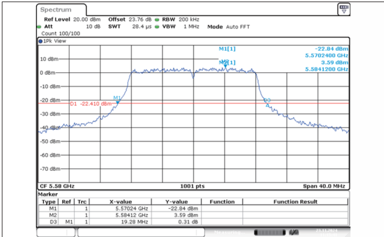
11A-Ant1-5580
