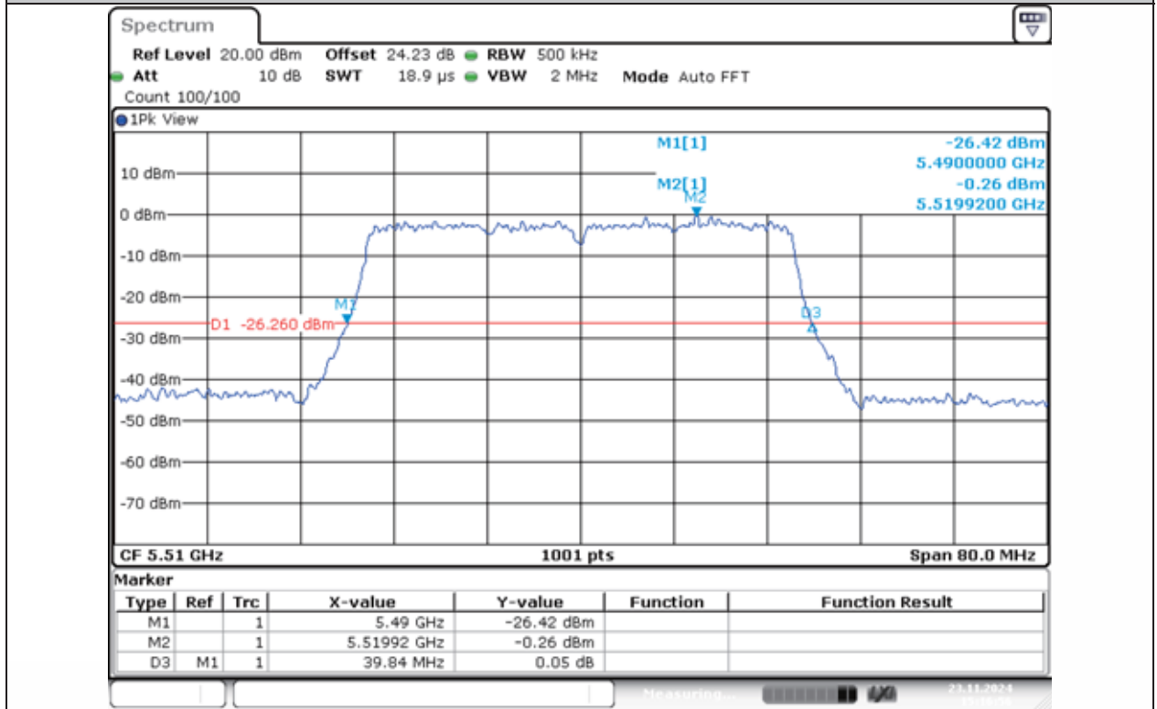
11N40MIMO-Ant1-5510
