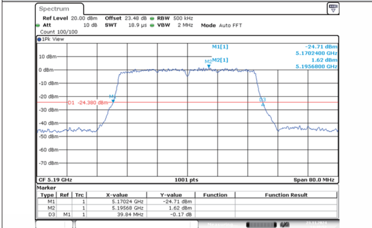
11N40MIMO-Ant1-5190
