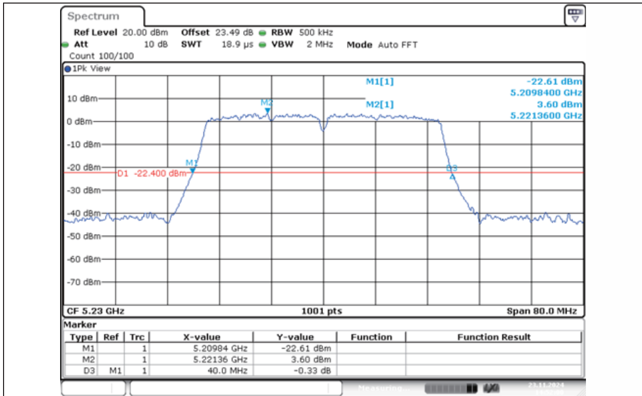
11N40MIMO-Ant1-5230
