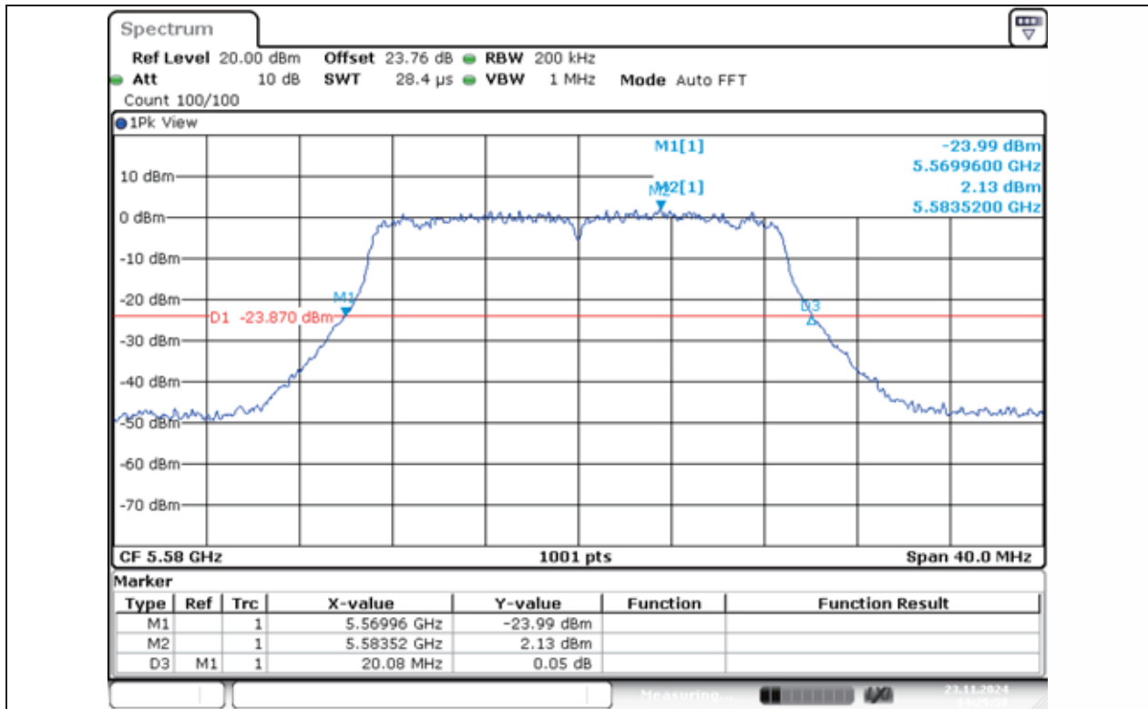
11N20MIMO-Ant1-5580
