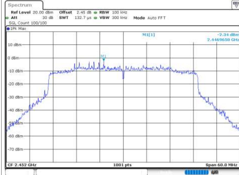
Band Edge NVNT ax40 2452MHz Ant2 Ref
