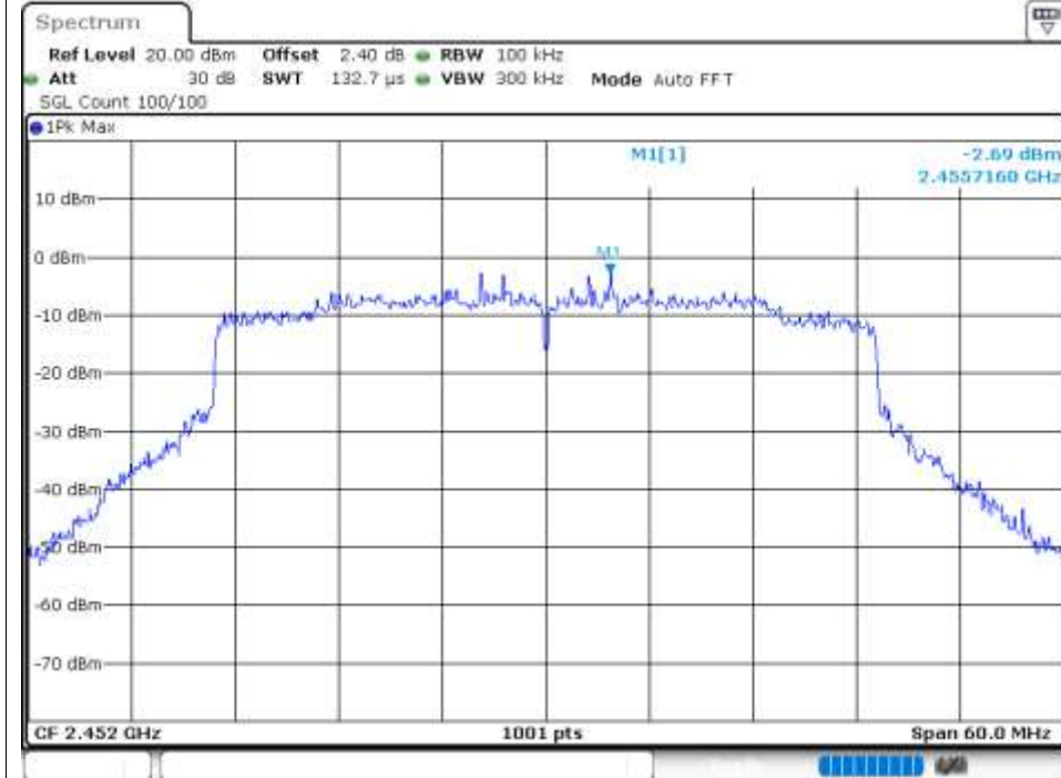
Band Edge NVNT ax40 2452MHz Ant1 Ref
