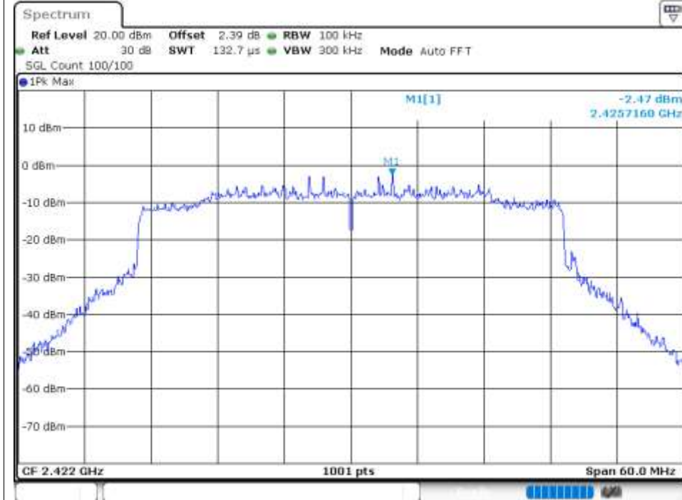
Band Edge NVNT ax40 2422MHz Ant1 Ref
