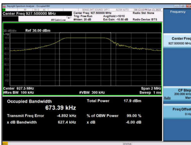
6dB EBW: 927.5MHz
