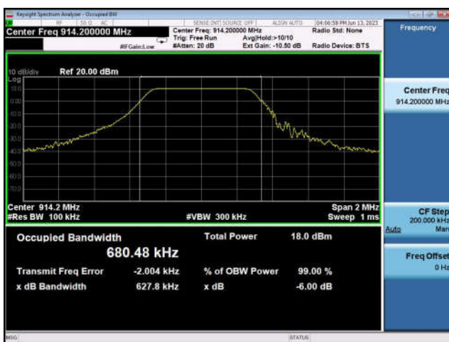
6dB EBW: 914.2MHz
