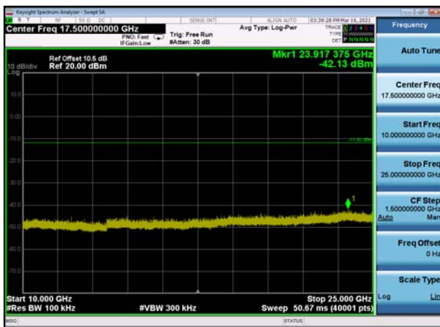
,Plot 5,10000MHz~25000MHz-802.11b ,2462MHz
