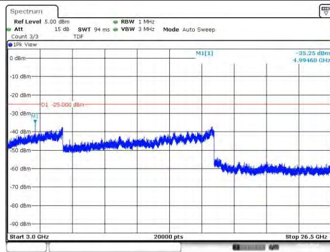
Band41-5MHz-QPSK-39675-25RB#0-Range3:3000~26500MHz
