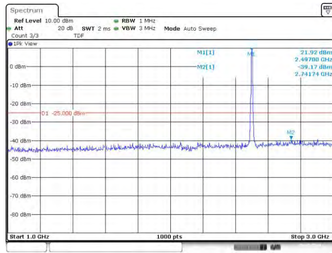
Band41-5MHz-QPSK-39675-25RB#0-Range2:1000~3000MHz
