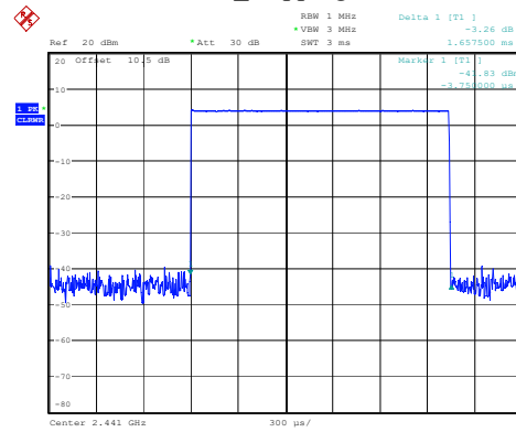
DH3_Hopping 1.658ms
