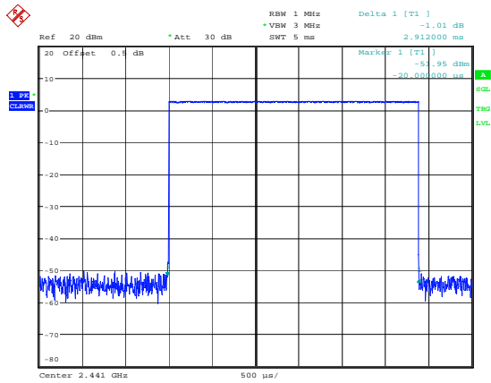
DH5_Hopping 2.912ms
