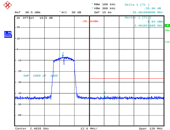
802.11n20_2462MHz
