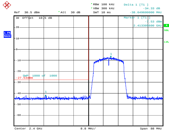
802.11n20_2412MHz
