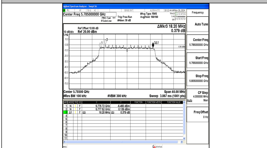
11AX20MIMO-Ant1-5785-PASS
