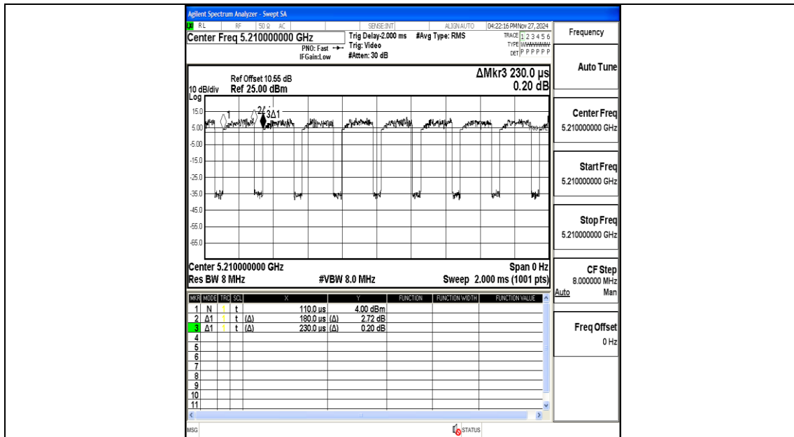
NTNV-11AX80MIMO-Ant1-5210
