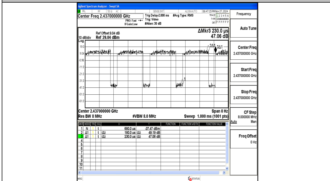
NTNV-11AX40MIMO-Ant2-2437
