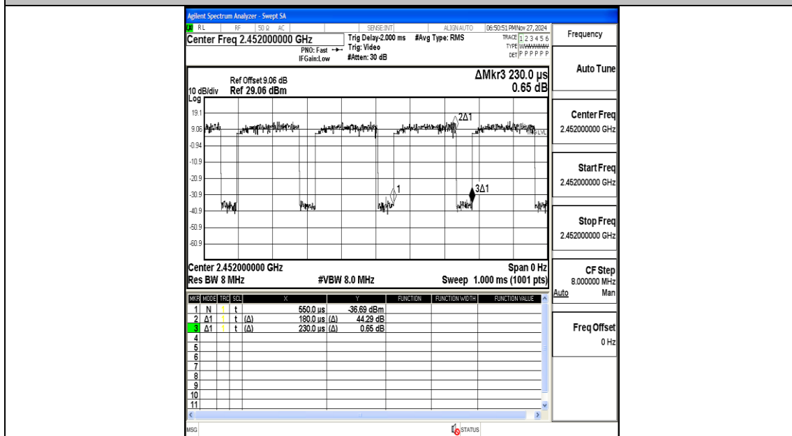
NTNV-11AX40MIMO-Ant1-2452
