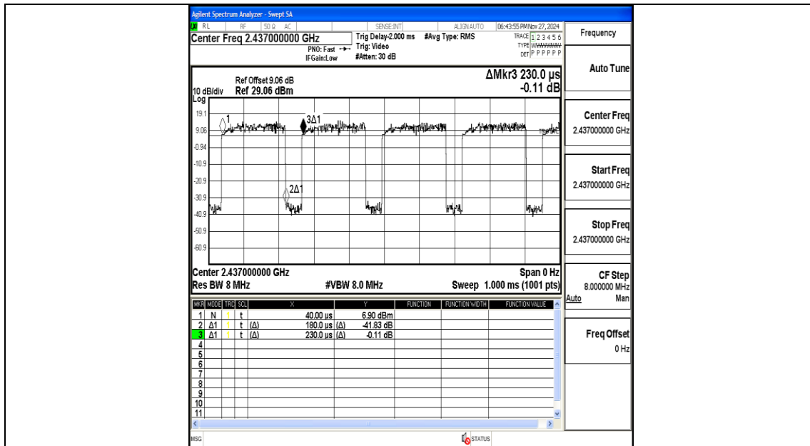
NTNV-11AX40MIMO-Ant1-2437
