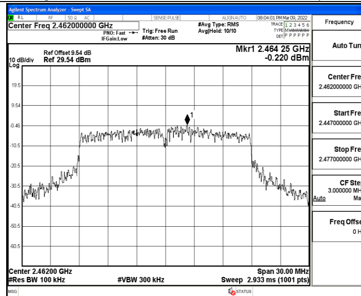
11N20MIMO_Ant2_2462_30~1000
