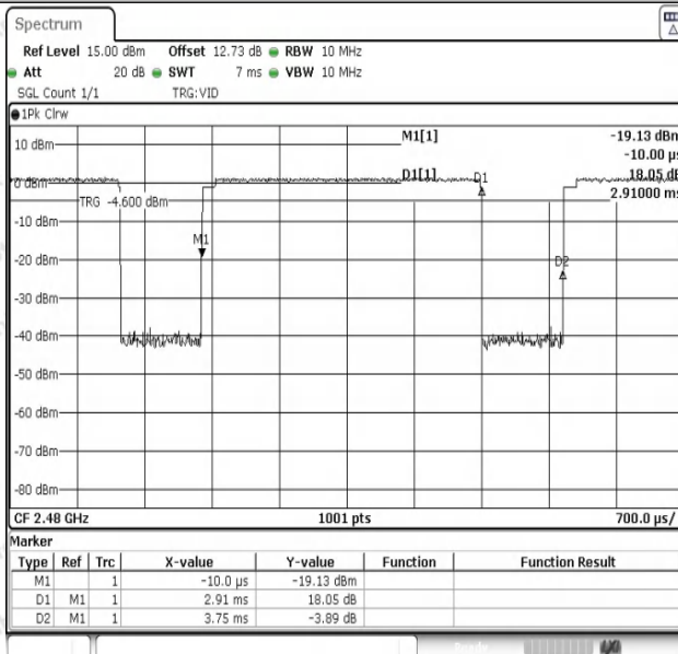
NTNV-2DH5-Ant1-2480
