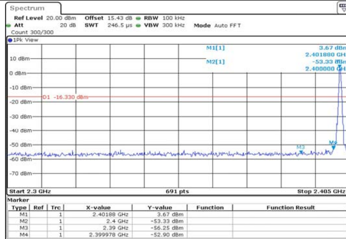
DH1_Ant1_Low_2402
