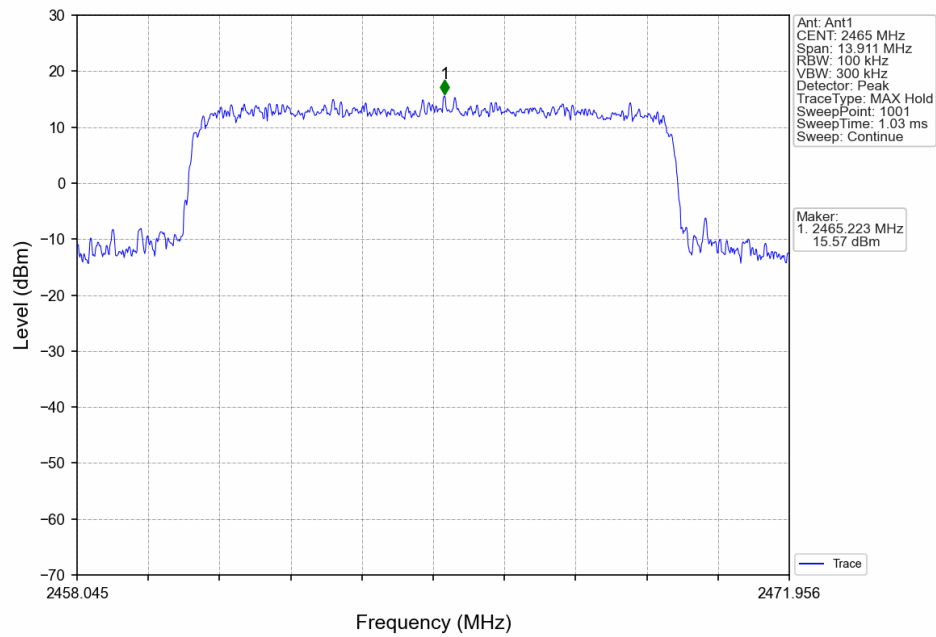
Slot10_HCH_2465MHz_Ant1_NTNV
