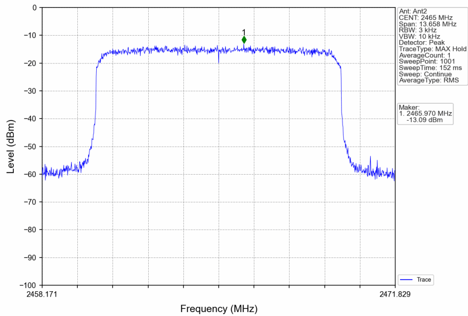
Slot10_HCH_2465MHz_MIMO_NTNV
