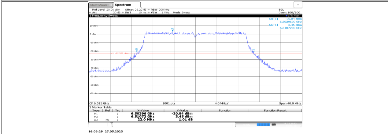
11AX20MIMO_Ant1_6515
