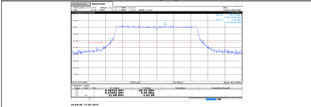
11AX20MIMO_Ant3_6475
