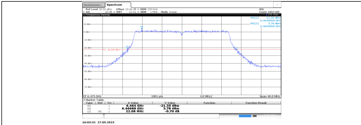
11AX20MIMO_Ant1_6475
