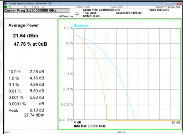
Band 7_1_Q16_Middle
