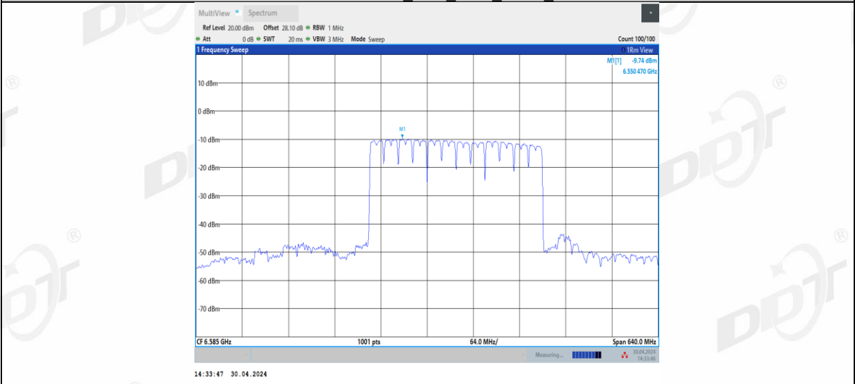
11BE320MIMO_Ant3_6585_3*996_2
