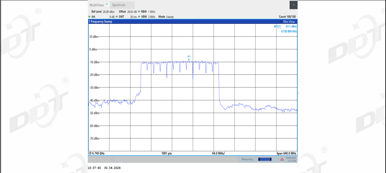
11BE320MIMO_Ant3_6745_2*996+484_7
