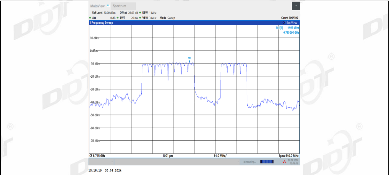
11BE320MIMO_Ant2_6745_3*996_4
