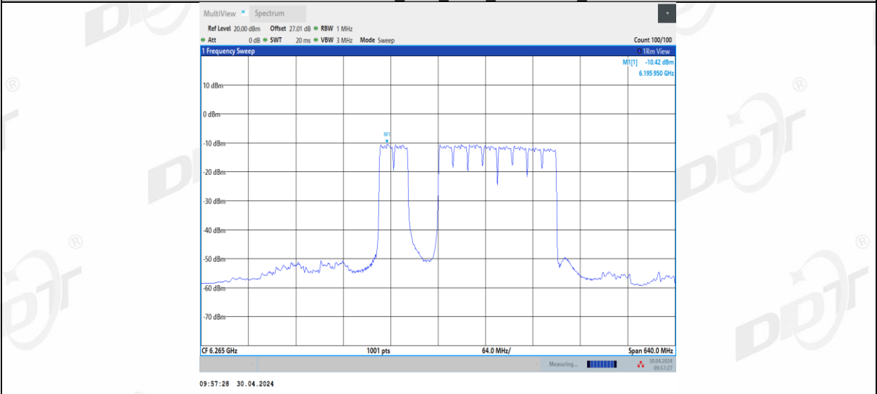
11BE320MIMO_Ant2_6265_2*996+484_9
