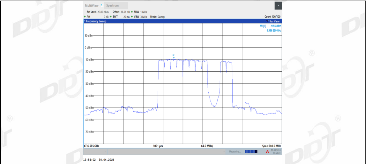
11BE320MIMO_Ant3_6585_2*996+484_12
