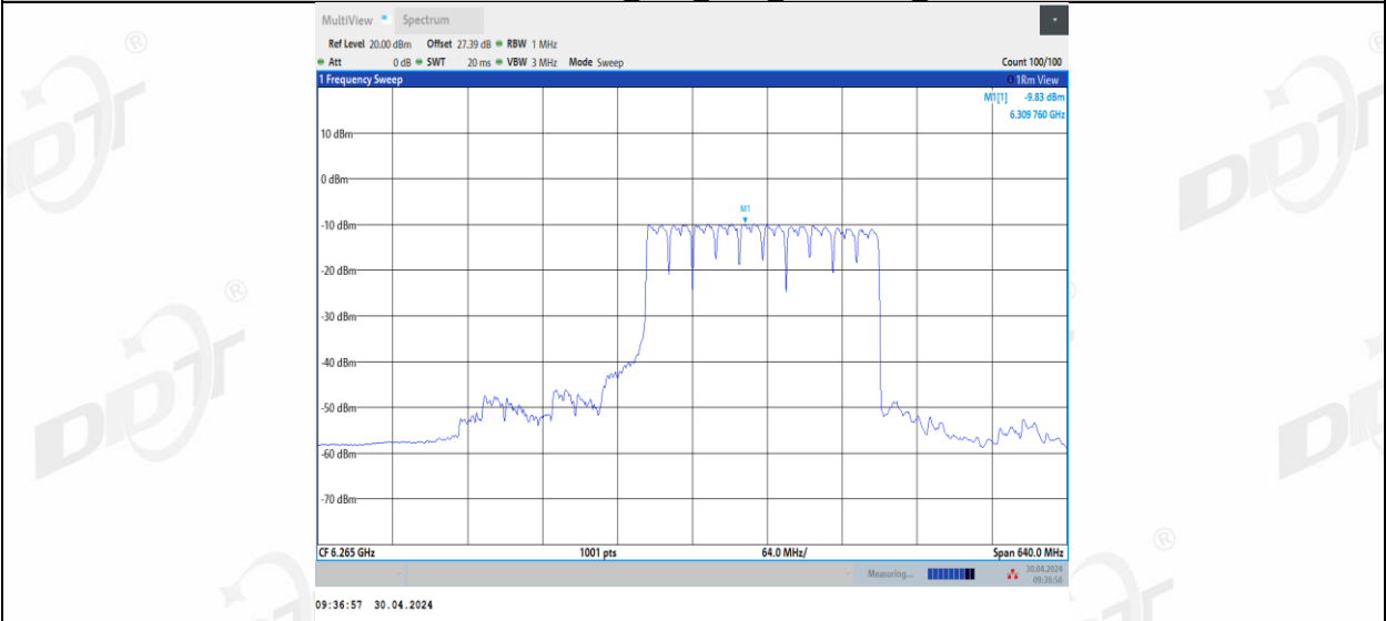
11BE320MIMO_Ant2_6265_2*996+484_8
