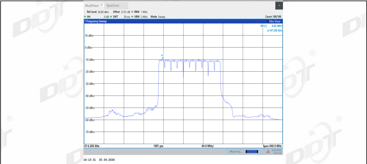
11BE320MIMO_Ant2_6265_3*996_1
