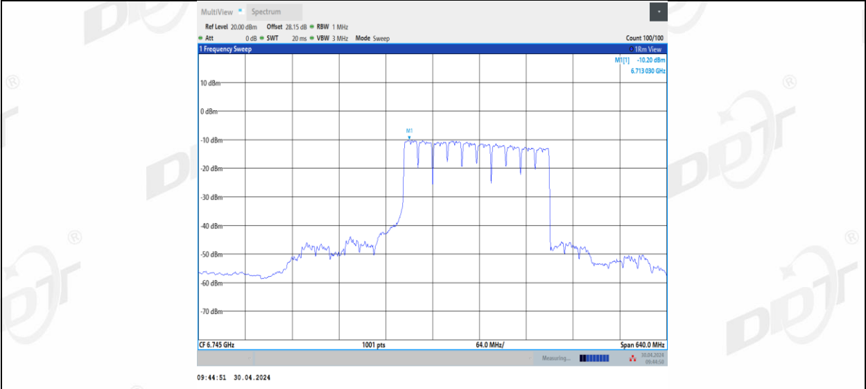
11BE320MIMO_Ant3_6745_2*996+484_8
