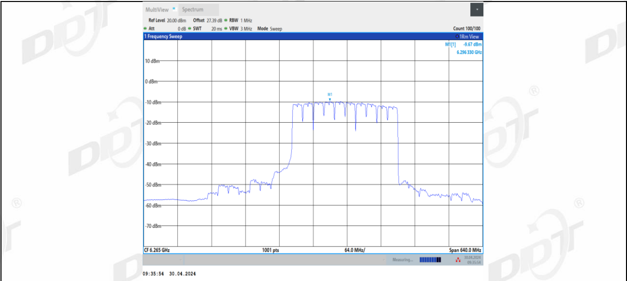
11BE320MIMO_Ant1_6265_2*996+484_8
