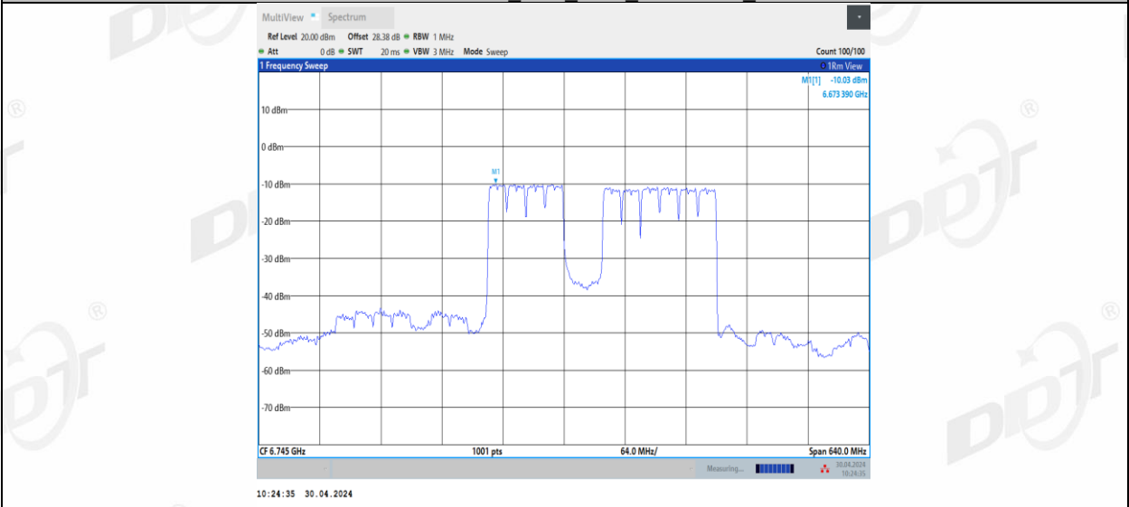
11BE320MIMO_Ant1_6745_2*996+484_10
