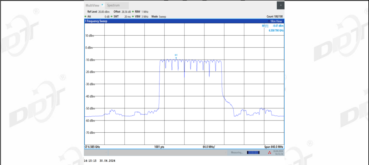
11BE320MIMO_Ant3_6585_3*996_1
