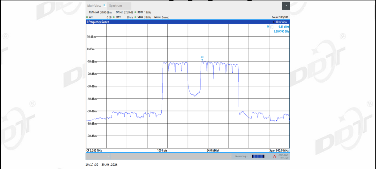
11BE320MIMO_Ant1_6265_2*996+484_10
