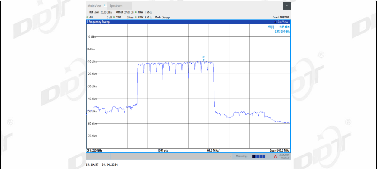
11BE320MIMO_Ant2_6265_2*996+484_7
