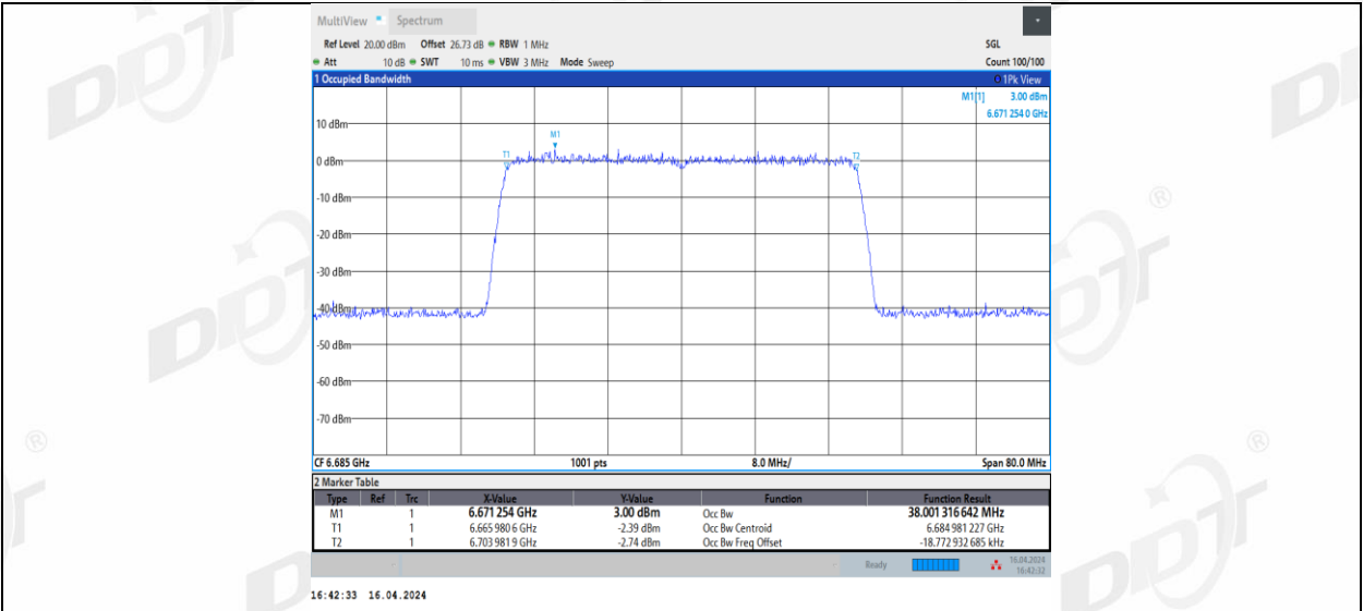
11AX40MIMO_Ant2_6685
