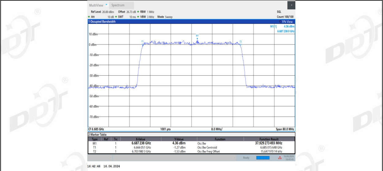
11AX40MIMO_Ant3_6685
