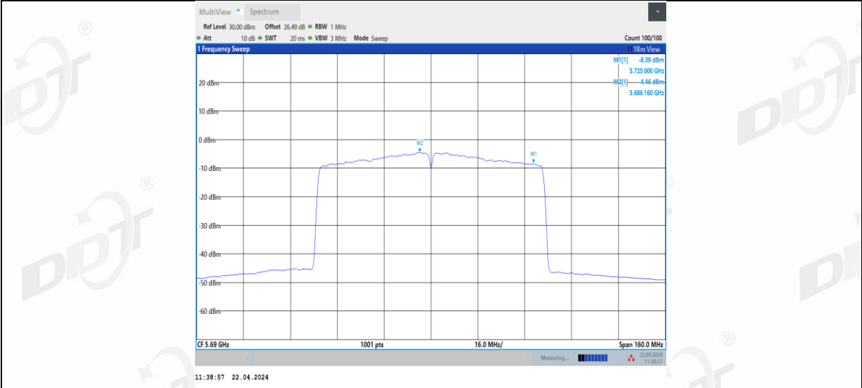
11AC80MIMO_Ant3_5690_UNII-2C
