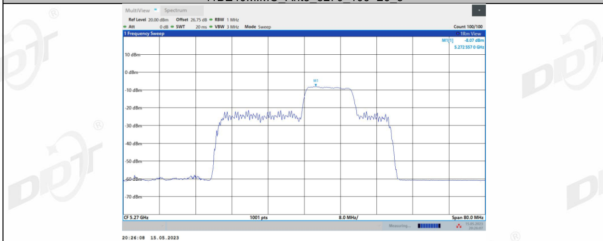
11BE40MIMO_Ant3_5270_106+26_4
