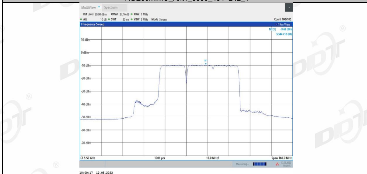
11BE80MIMO Ant1 5530 484+242 2
