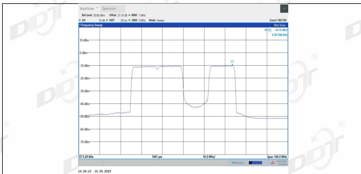
11BE80MIMO Ant4 5290 484+242 4
