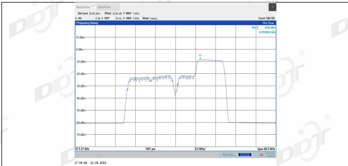
11BE40MIMO_Ant3_5270_106+26_3
