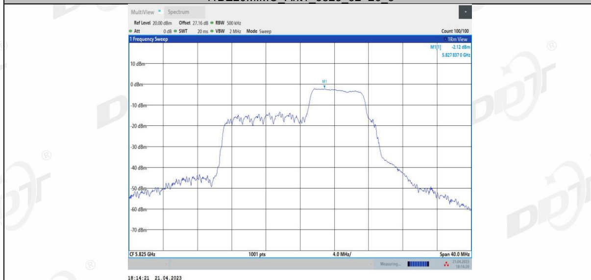
11BE20MIMO Ant1 5825 106+26 1
