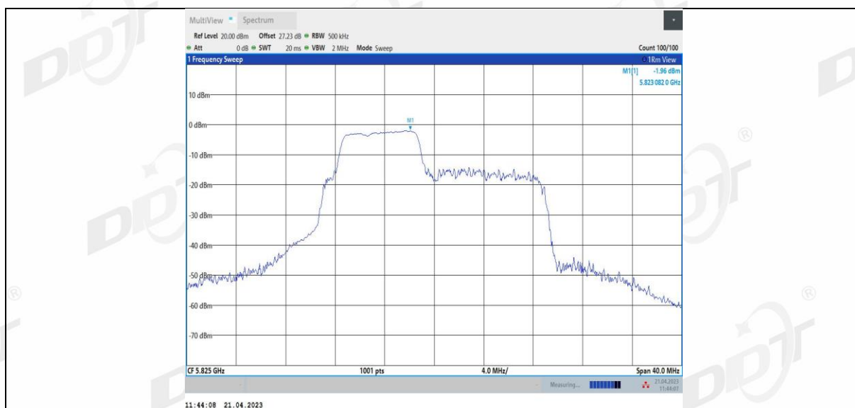
11BE20MIMO Ant1 5825 52+26 2
