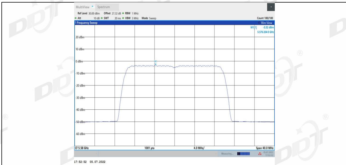
11AX20MIMO_Ant2_5580
