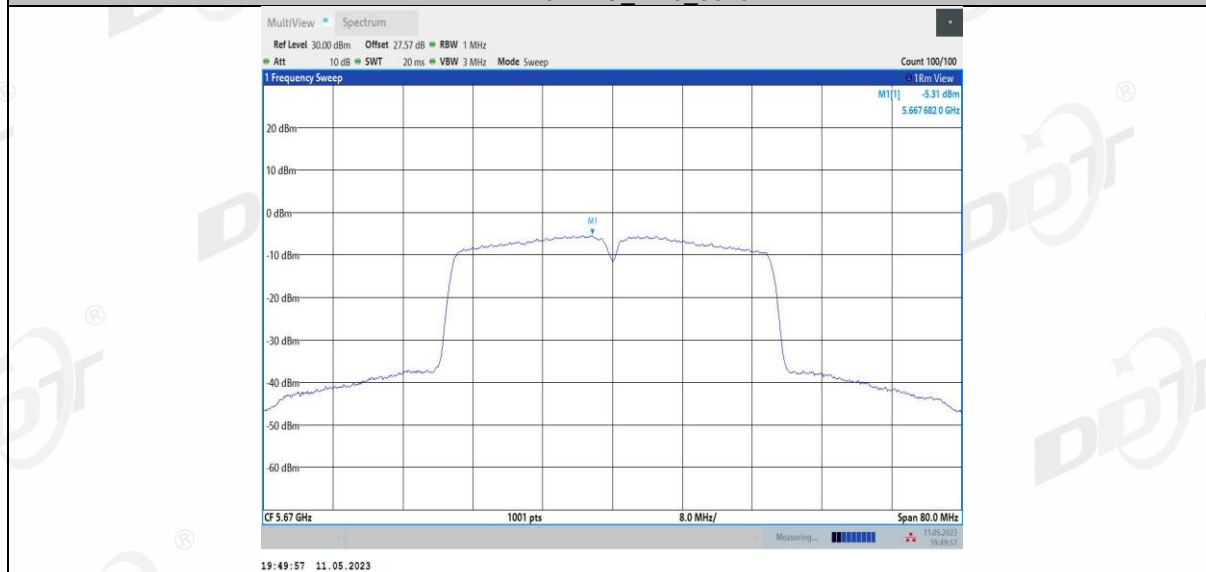
11AX40MIMO_Ant4_5670
