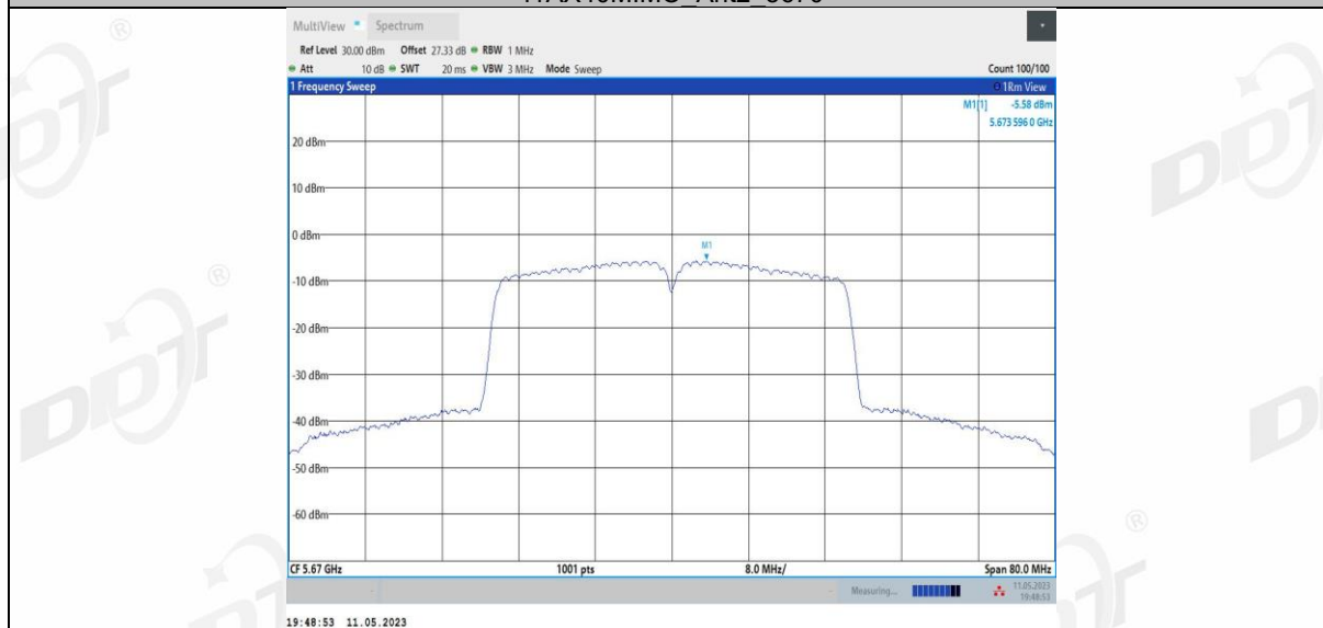
11AX40MIMO_Ant3_5670
