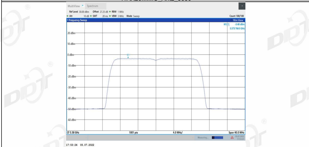
11AX20MIMO_Ant3_5580
