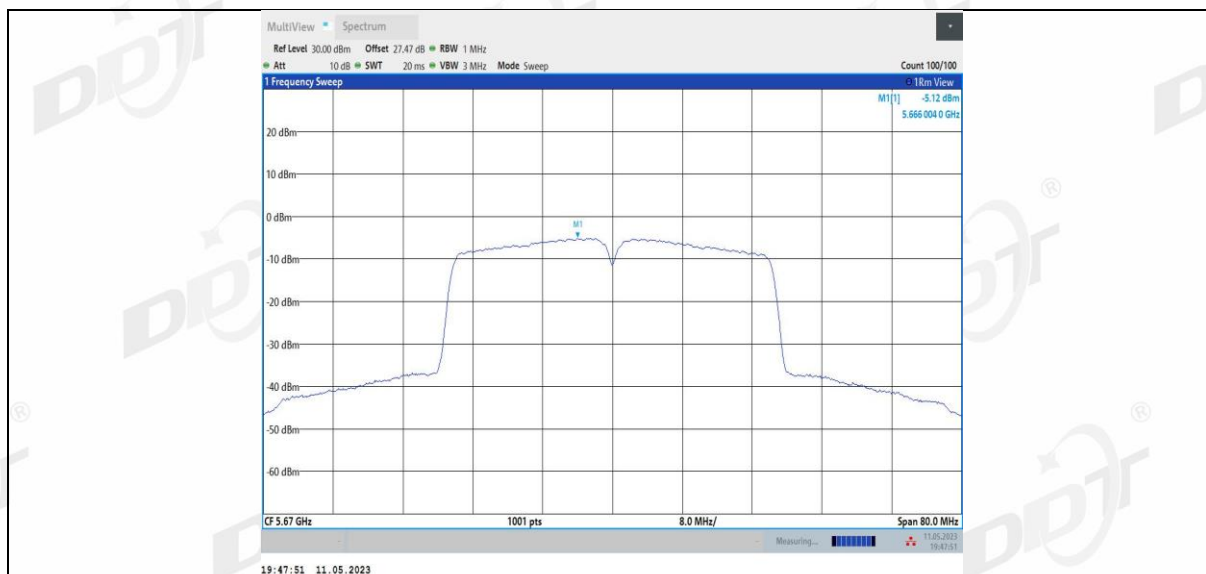
11AX40MIMO_Ant2_5670
