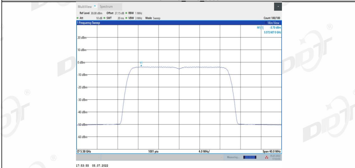
11AX20MIMO_Ant4_5580
