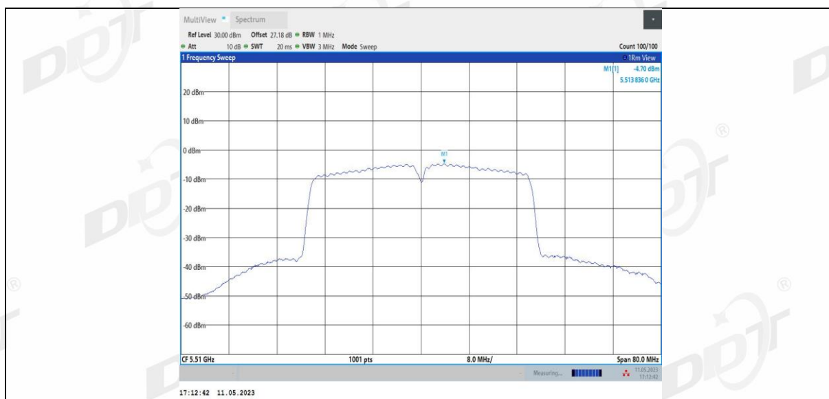
11AC40MIMO_Ant2_5510
