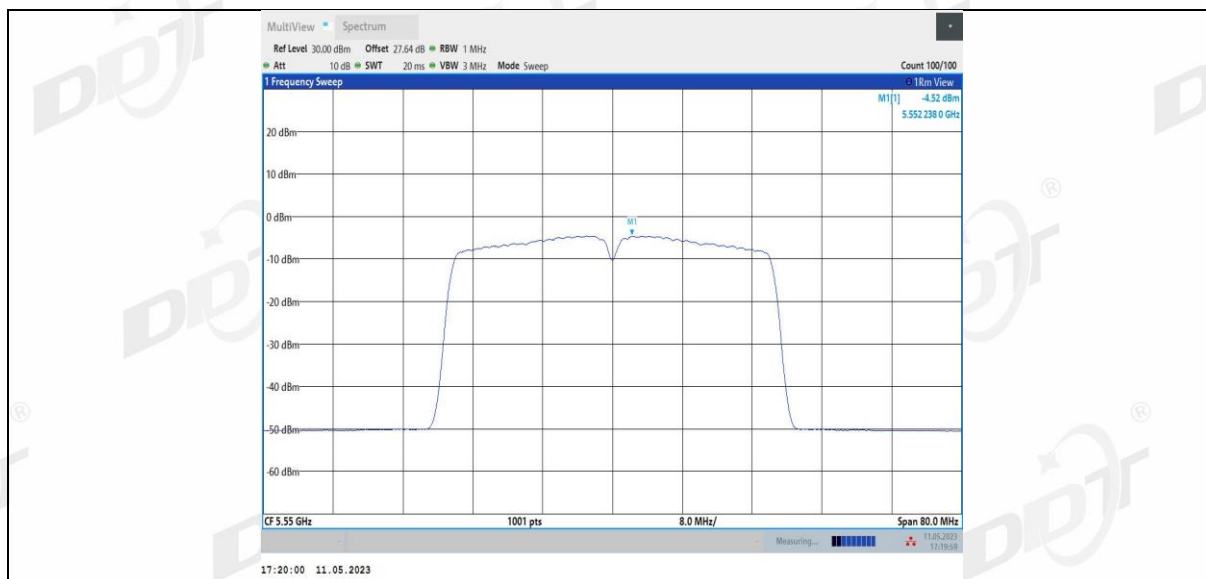
11AC40MIMO_Ant4_5550
