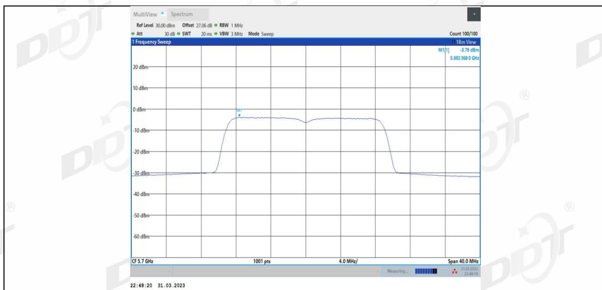
11N20MIMO Ant4 5700
