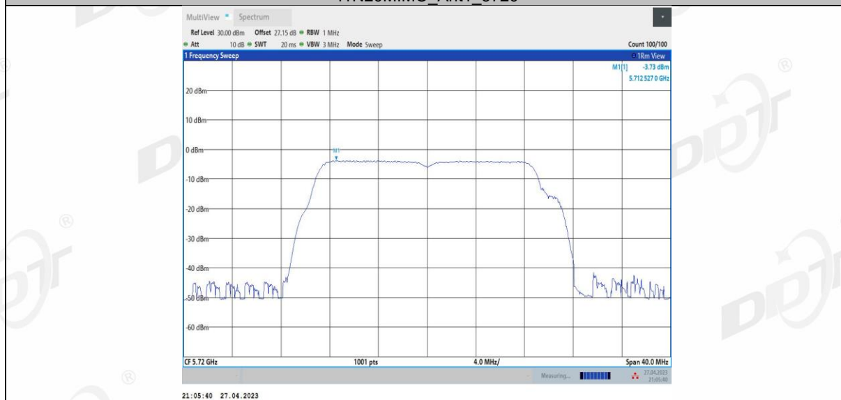
11N20MIMO Ant2 5720
