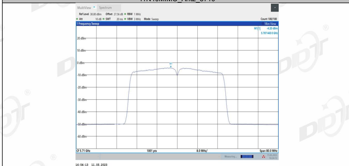
11N40MIMO Ant3 5710
