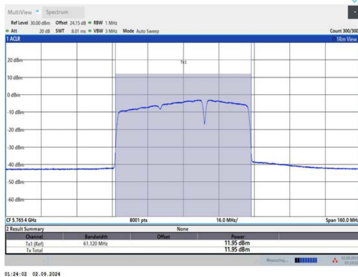
11BE80MIMO_Ant3_5775_484+242_OFDMA_1
