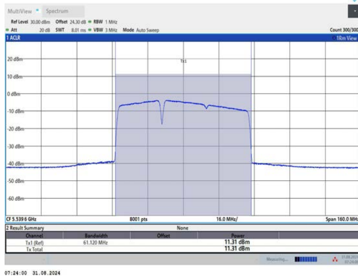
11BE80MIMO_Ant3_5530_484+242_OFDMA_2
