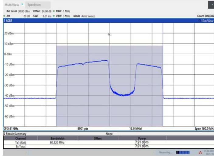
11BE80MIMO_Ant1_5610_484+242_OFDMA_3
