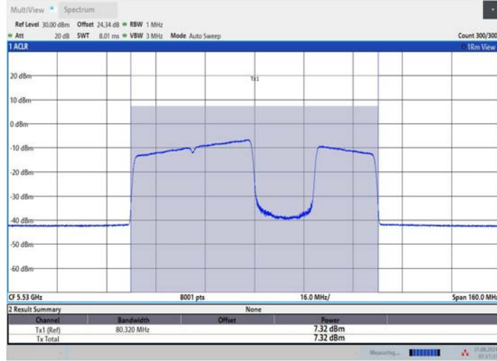
11BE80MIMO_Ant3_5530_484+242_OFDMA_3
