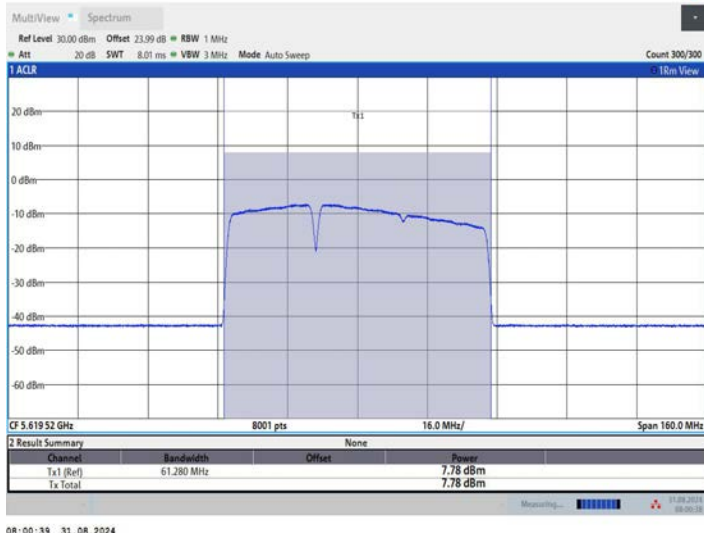
11BE80MIMO_Ant3_5610_484+242_OFDMA_1
