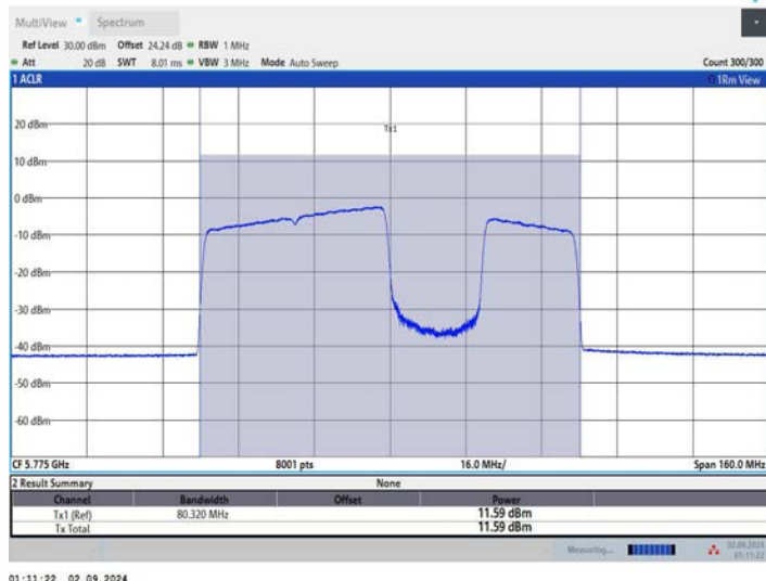
11BE80MIMO_Ant1_5775_484+242_OFDMA_4
