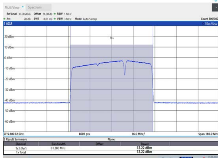
11BE80MIMO_Ant2_5610_484+242_OFDMA_1
