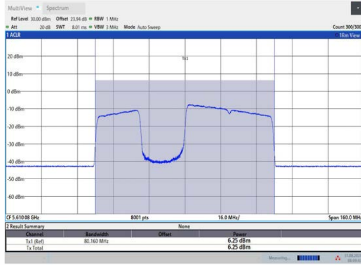
11BE80MIMO_Ant2_5610_484+242_OFDMA_2
