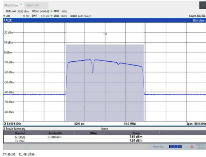
11BE80MIMO_Ant1_5610_484+242_OFDMA_1
