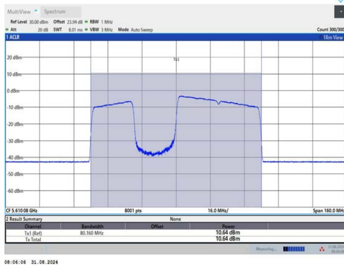
11BE80MIMO_Ant2_5610_484+242_OFDMA_3
