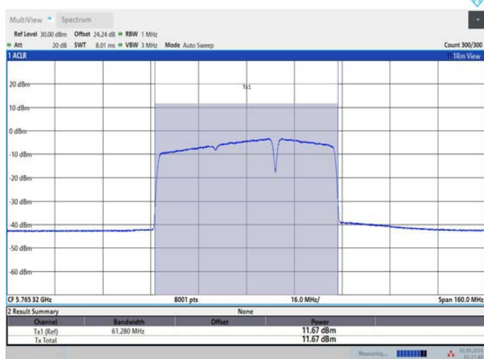
11BE80MIMO_Ant2_5775_484+242_OFDMA_1
