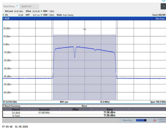
11BE80MIMO_Ant1_5610_484+242_OFDMA_2
