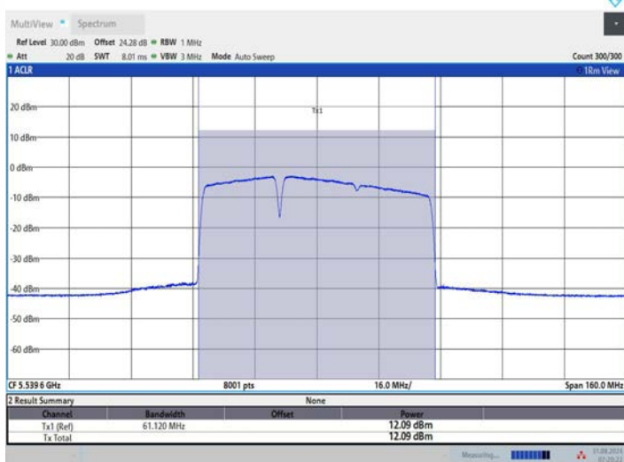
11BE80MIMO_Ant1_5530_484+242_OFDMA_2
