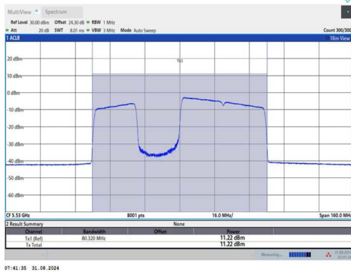
11BE80MIMO_Ant3_5530_484+242_OFDMA_3
