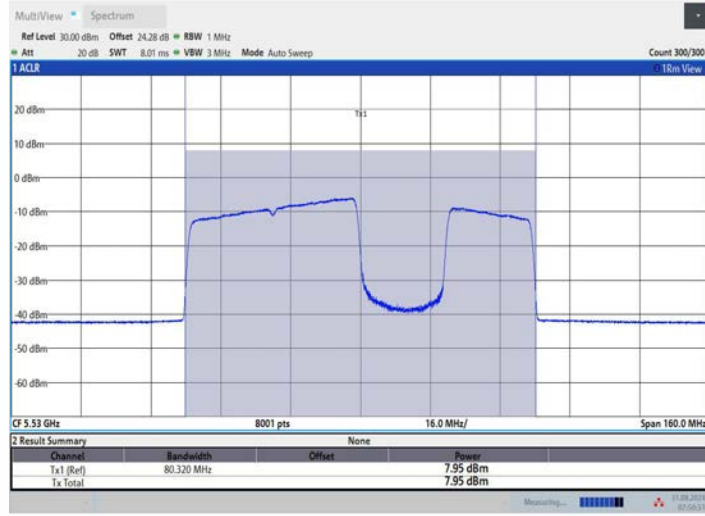
11BE80MIMO_Ant1_5530_484+242_OFDMA_3
