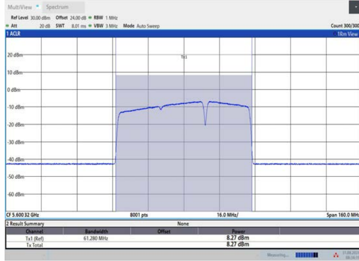
11BE80MIMO_Ant1_5610_484+242_OFDMA_4
