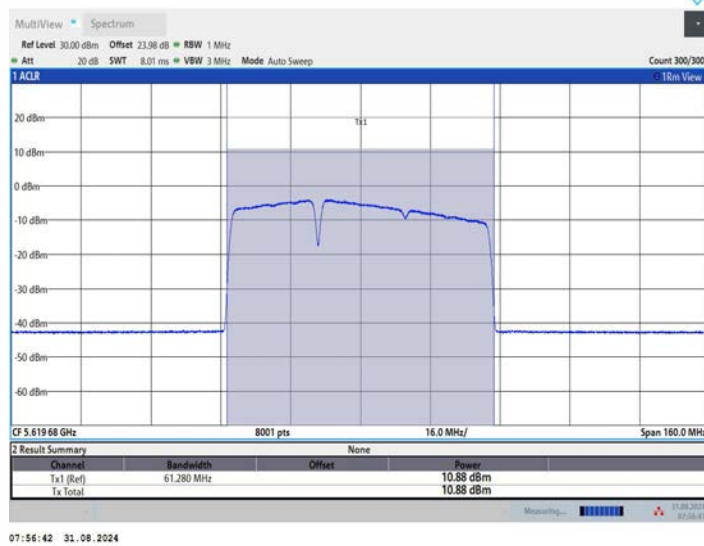
11BE80MIMO_Ant2_5610_484+242_OFDMA_2
