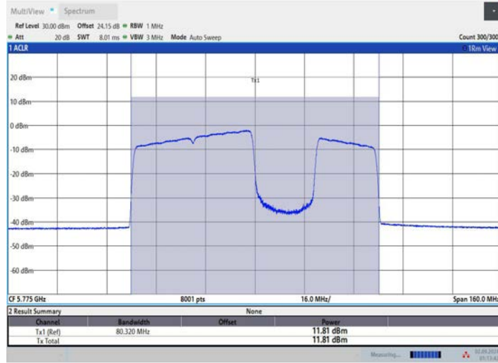
11BE80MIMO_Ant2_5775_484+242_OFDMA_4
