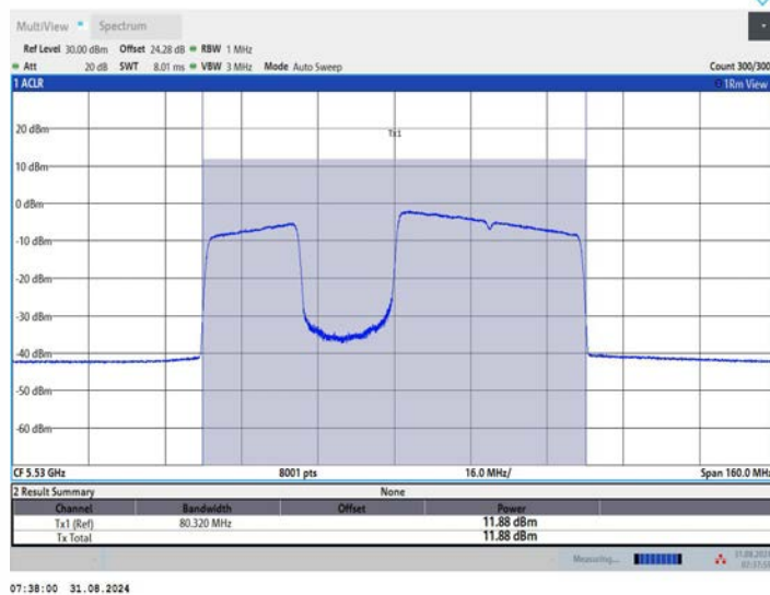
11BE80MIMO_Ant1_5530_484+242_OFDMA_3
