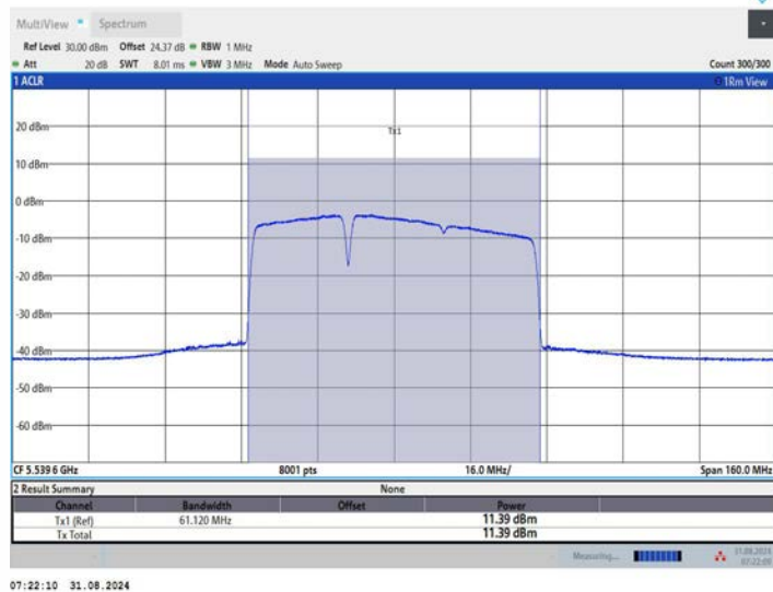
11BE80MIMO_Ant2_5530_484+242_OFDMA_2
