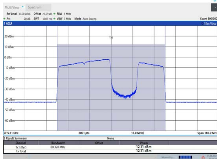
11BE80MIMO_Ant3_5610_484+242_OFDMA_4
