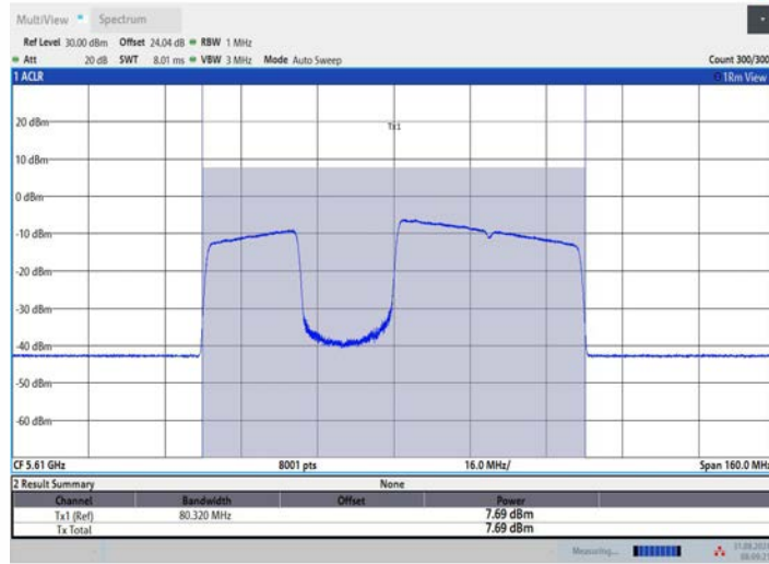
11BE80MIMO_Ant1_5610_484+242_OFDMA_2
