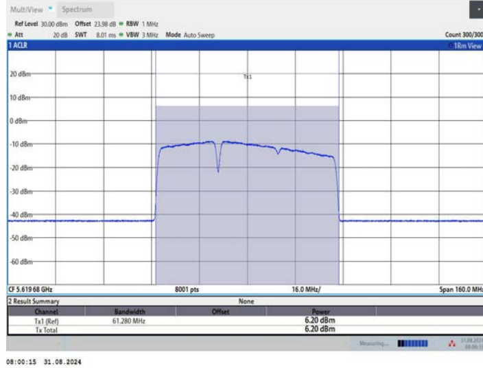
11BE80MIMO_Ant2_5610_484+242_OFDMA_1
