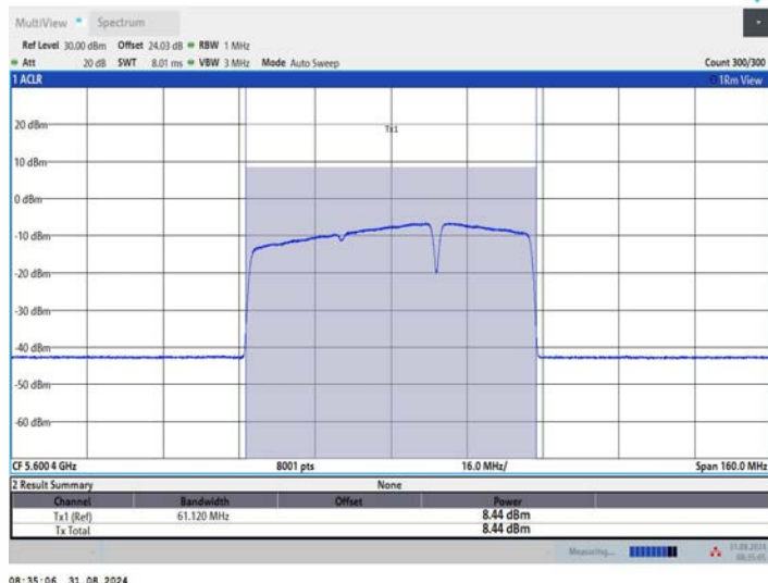
11BE80MIMO_Ant3_5610_484+242_OFDMA_4
