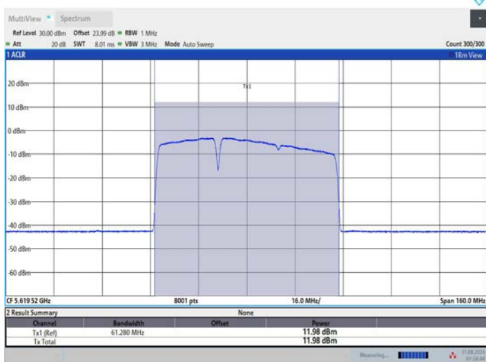
11BE80MIMO_Ant3_5610_484+242_OFDMA_2
