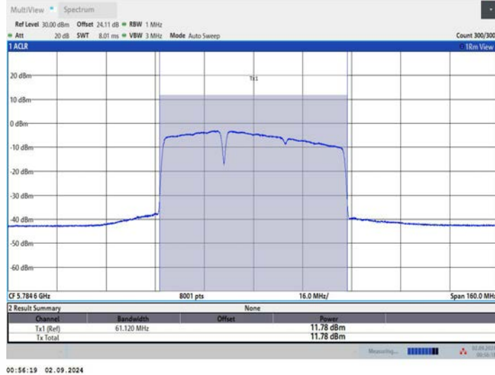
11BE80MIMO_Ant2_5775_484+242_OFDMA_2
