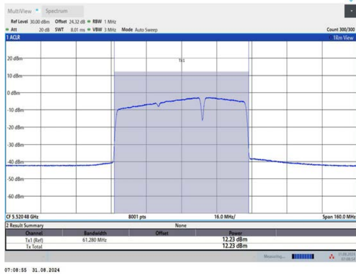
11BE80MIMO_Ant2_5530_484+242_OFDMA_1
