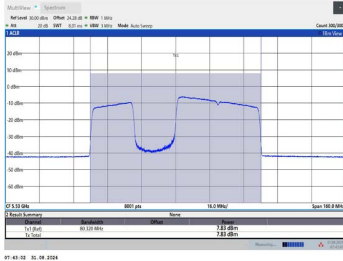
11BE80MIMO_Ant1_5530_484+242_OFDMA_2
