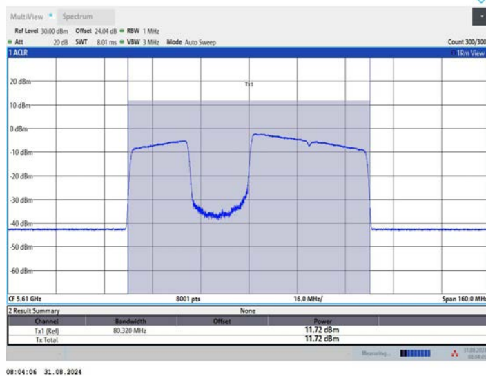
11BE80MIMO_Ant1_5610_484+242_OFDMA_3
