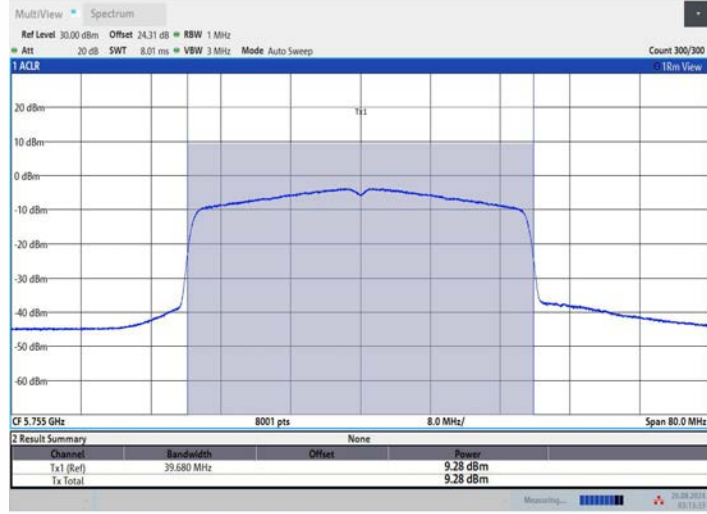
11AX40MIMO_Ant2_5755
