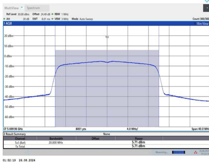
11AX20MIMO_Ant1_5700
