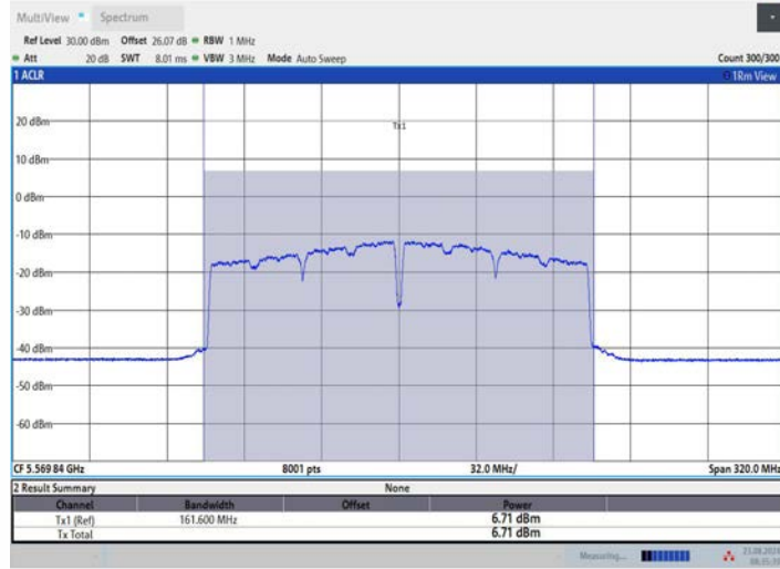
11AC160MIMO_Ant3_5570
