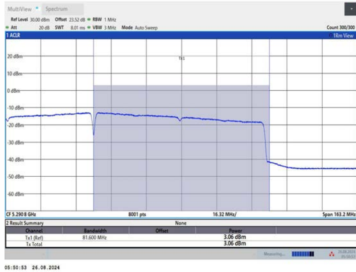
11AX160MIMO_Ant1_5250_UNII-2A
