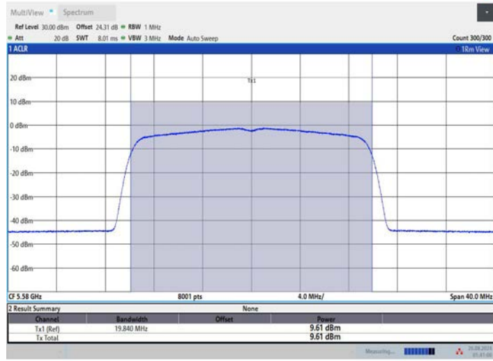
11AX20MIMO_Ant3_5580
