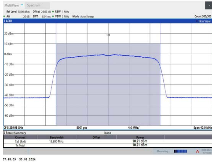
11BE20MIMO_Ant2_5240
