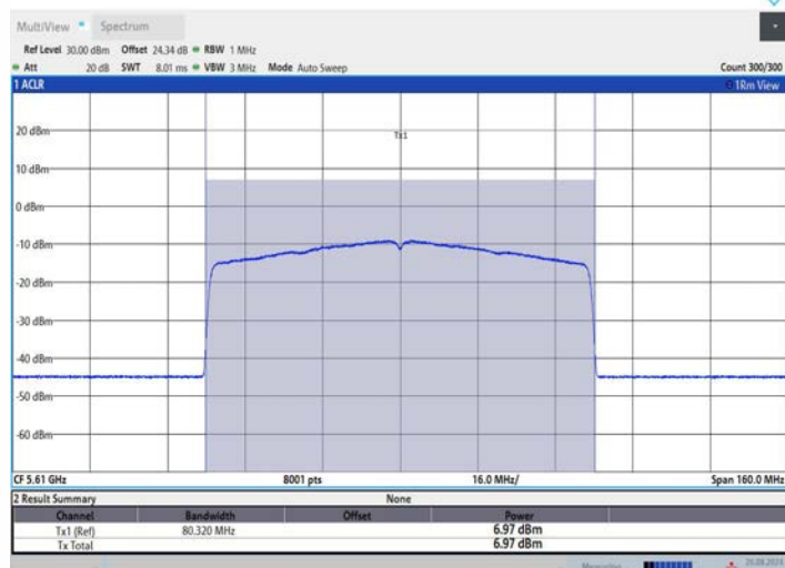
11AX80MIMO_Ant3_5610
