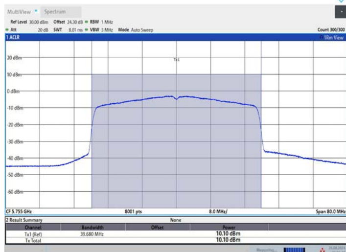
11AX40MIMO_Ant3_5755
