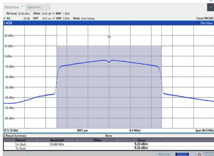
11AX40MIMO_Ant3_5190
