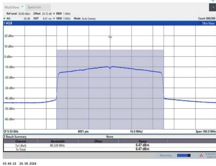
11AX80MIMO_Ant1_5530
