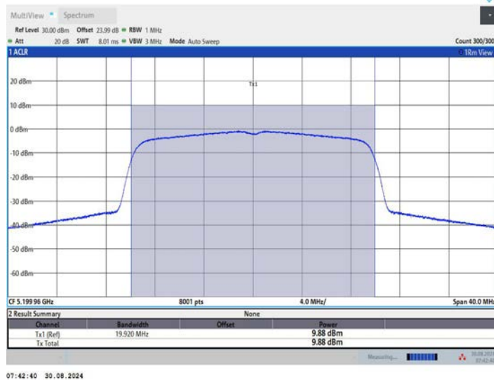
11BE20MIMO_Ant2_5200
