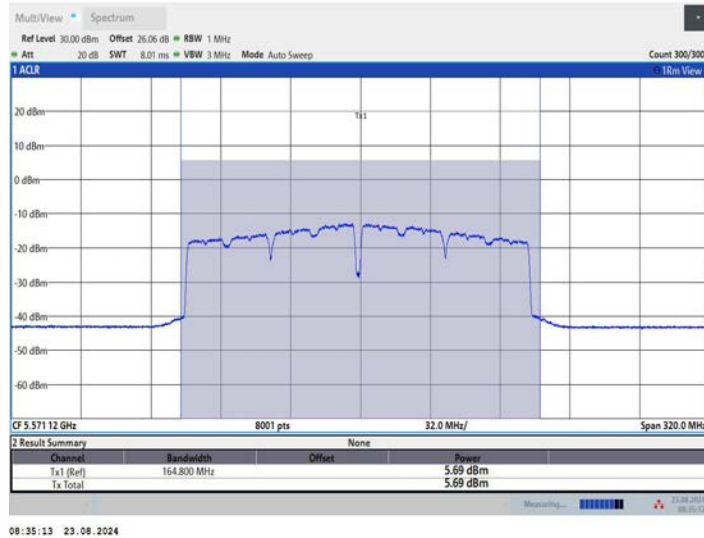
11AC160MIMO_Ant2_5570
