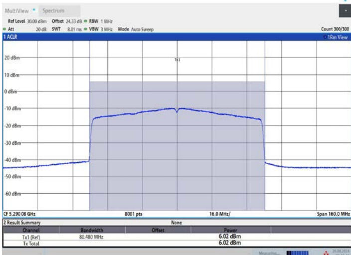
11AX80MIMO_Ant3_5290
