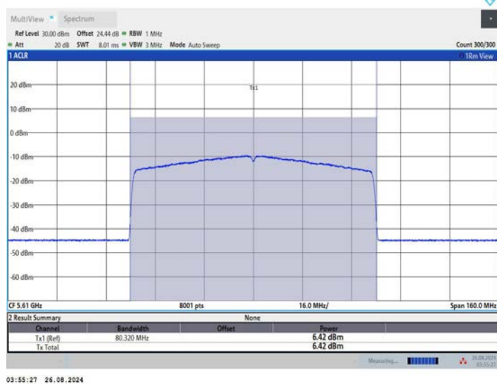
11AX80MIMO_Ant1_5610
