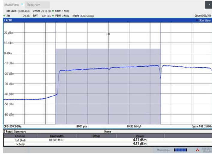
11AX160MIMO_Ant3_5250_UNII-1
