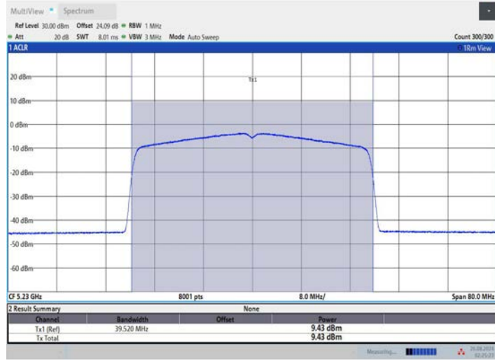
11AX40MIMO_Ant3_5230
