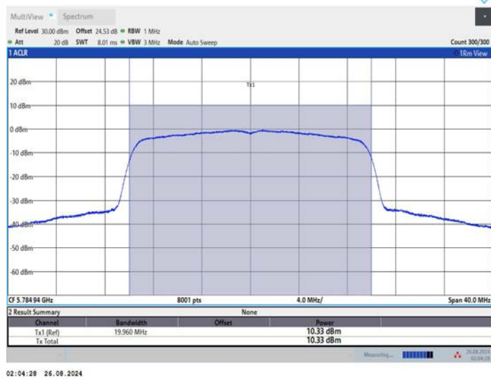
11AX20MIMO_Ant3_5785
