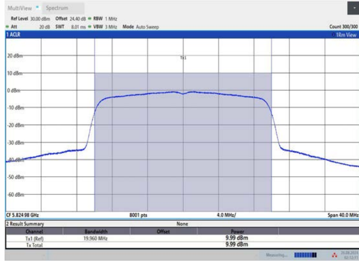
11AX20MIMO_Ant3_5825
