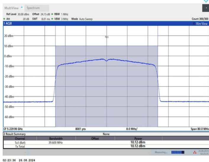
11AX40MIMO_Ant2_5230
