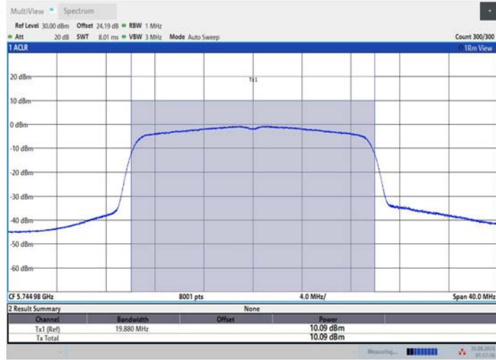
11AX20MIMO_Ant3_5745
