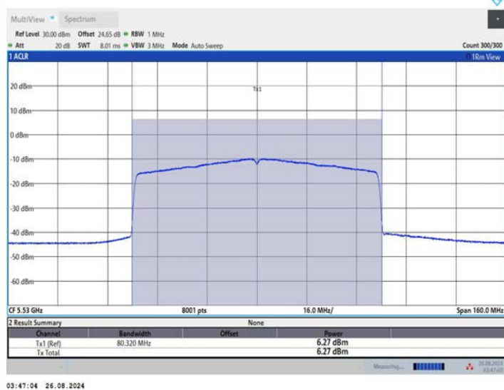
11AX80MIMO_Ant3_5530
