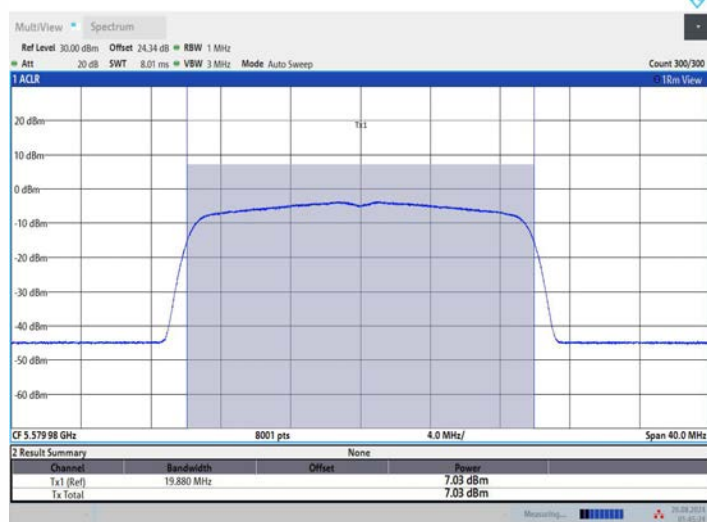
11AX20MIMO_Ant3_5580
