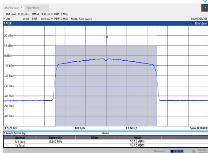
11AX40MIMO_Ant2_5270
