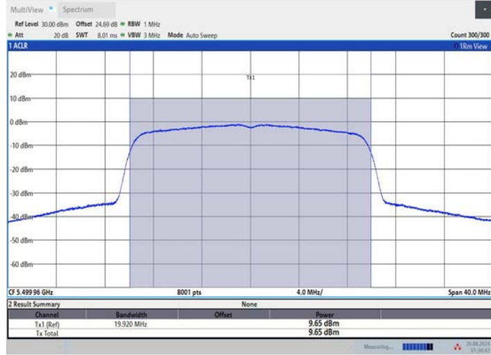
11AX20MIMO_Ant3_5500
