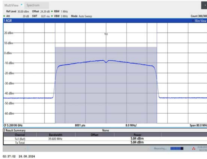
11AX40MIMO_Ant3_5270
