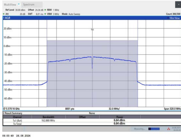
11AX160MIMO_Ant3_5570
