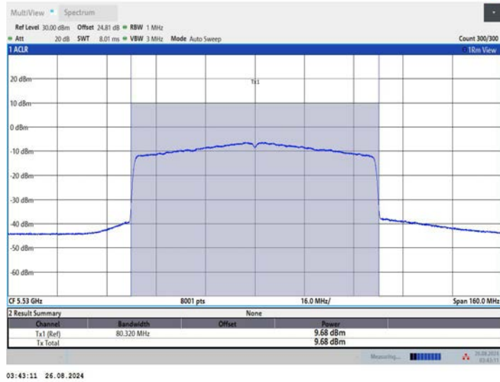
11AX80MIMO_Ant3_5530
