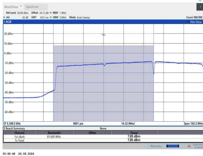
11AX160MIMO_Ant1_5250_UNII-2A
