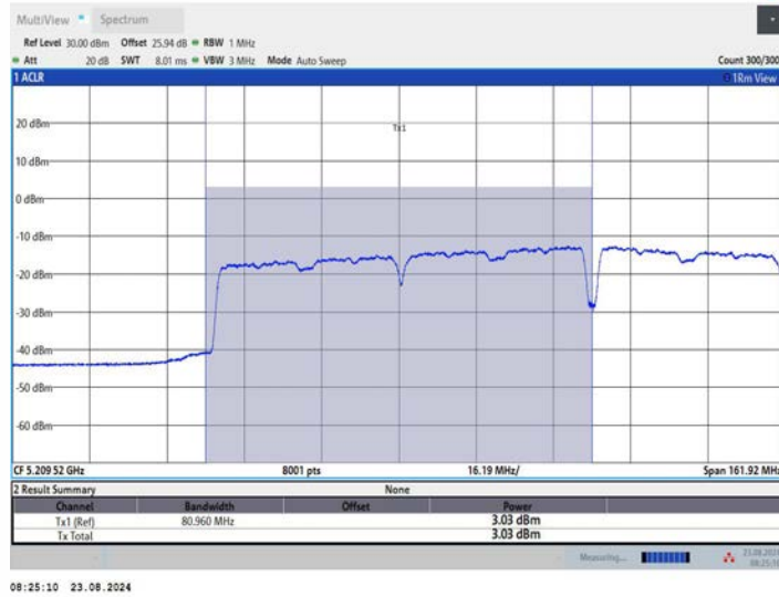
11AC160MIMO_Ant2_5250_UNII-1
