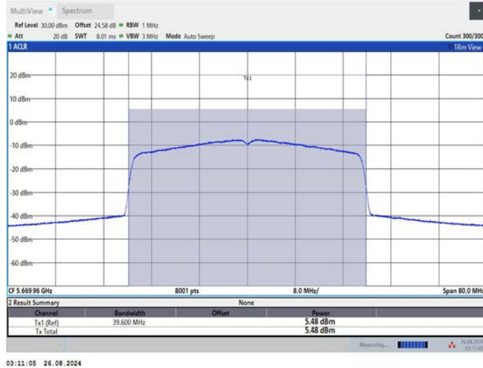
11AX40MIMO_Ant3_5670
