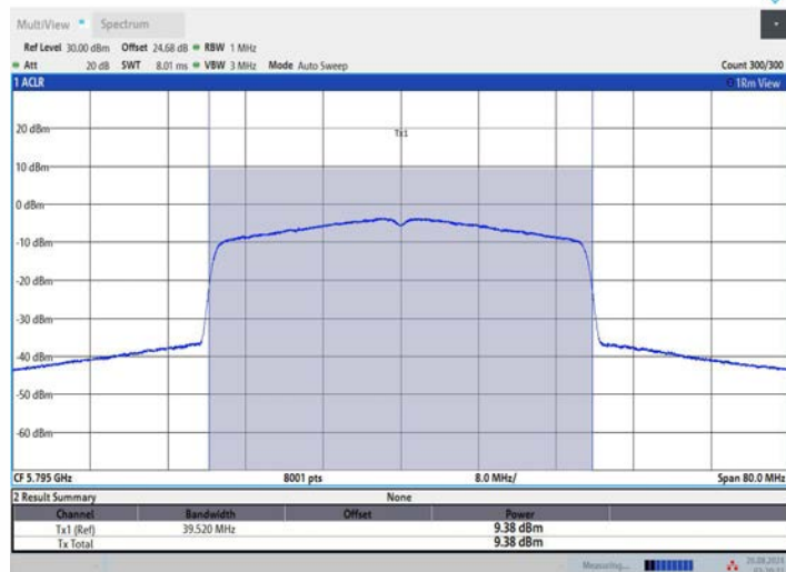
11AX40MIMO_Ant2_5795
