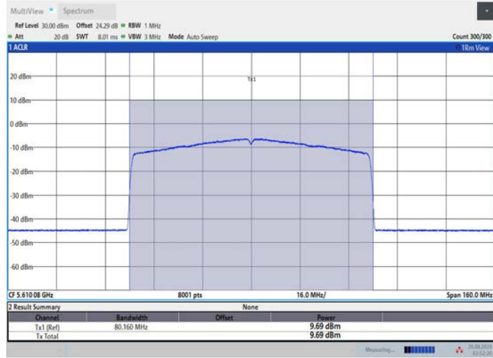
11AX80MIMO_Ant3_5610
