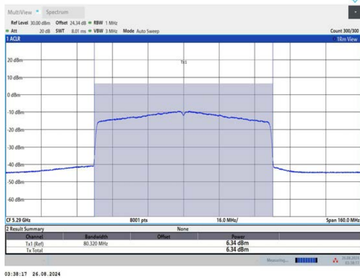
11AX80MIMO_Ant1_5290
