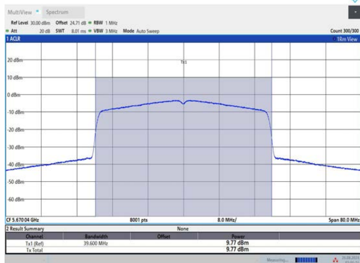
11AX40MIMO_Ant2_5670
