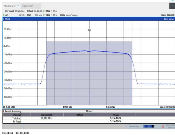
11AX20MIMO_Ant2_5580
