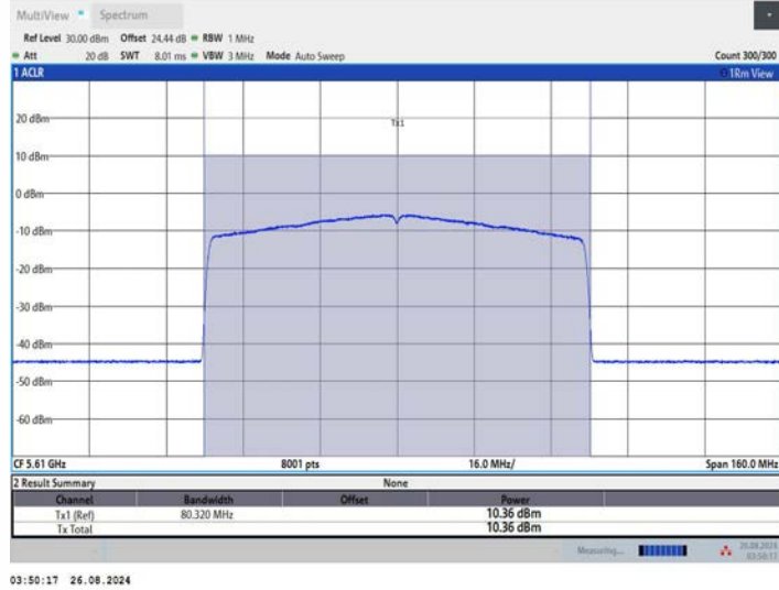
11AX80MIMO_Ant2_5610
