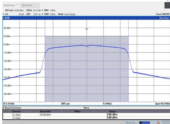
11AX20MIMO_Ant3_5180
