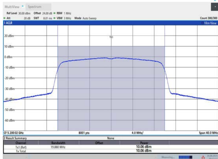
11AX20MIMO_Ant2_5200
