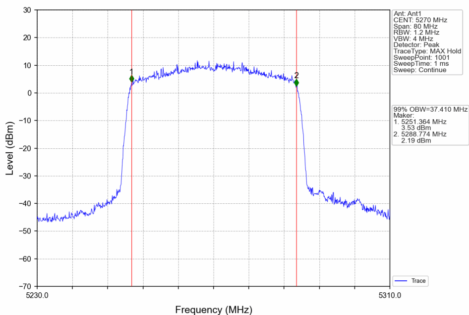
802.11ax(HEW40)_LCH_5270MHz_RU484_Left_Ant1_NTNV
