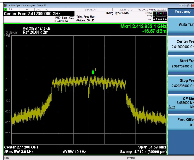
11G_Ant2_2412
