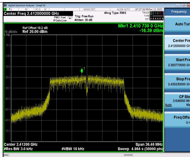
11N20MIMO_Ant2_2412
