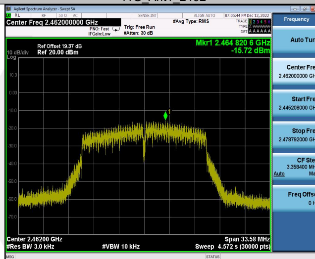
11G_Ant2_2462
