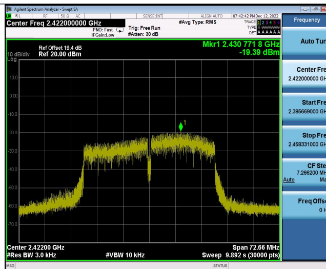
11N40MIMO_Ant2_2422
