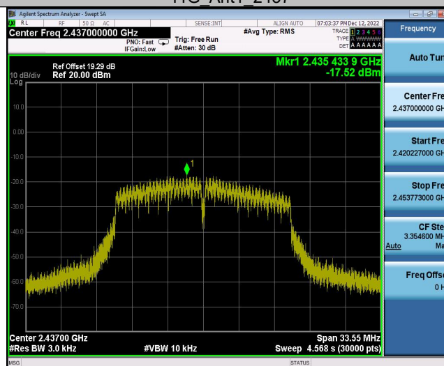
11G_Ant2_2437
