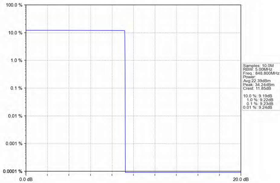
GSM850_GSM_HCH_848.8MHz_GSM_NTNV
