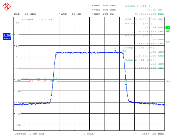
Band2-10MHz-16QAM-18900-50RB#0
